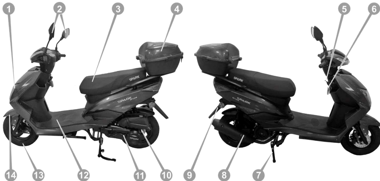
Рис.3.1. Основні вузли та агрегати
