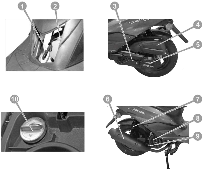
Рис. 3.4. Силовий агрегат
