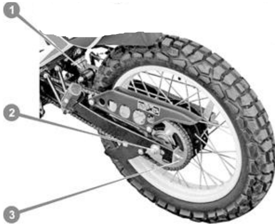
Рисунок 6.7. Ланцюгова передача і маятникова підвіска
