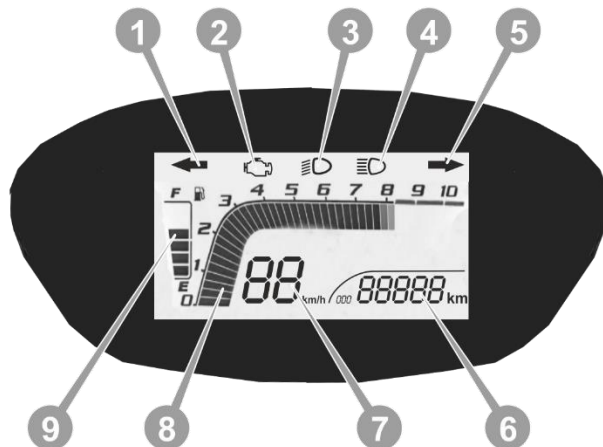
Рис. 3.2. Панель приладів
