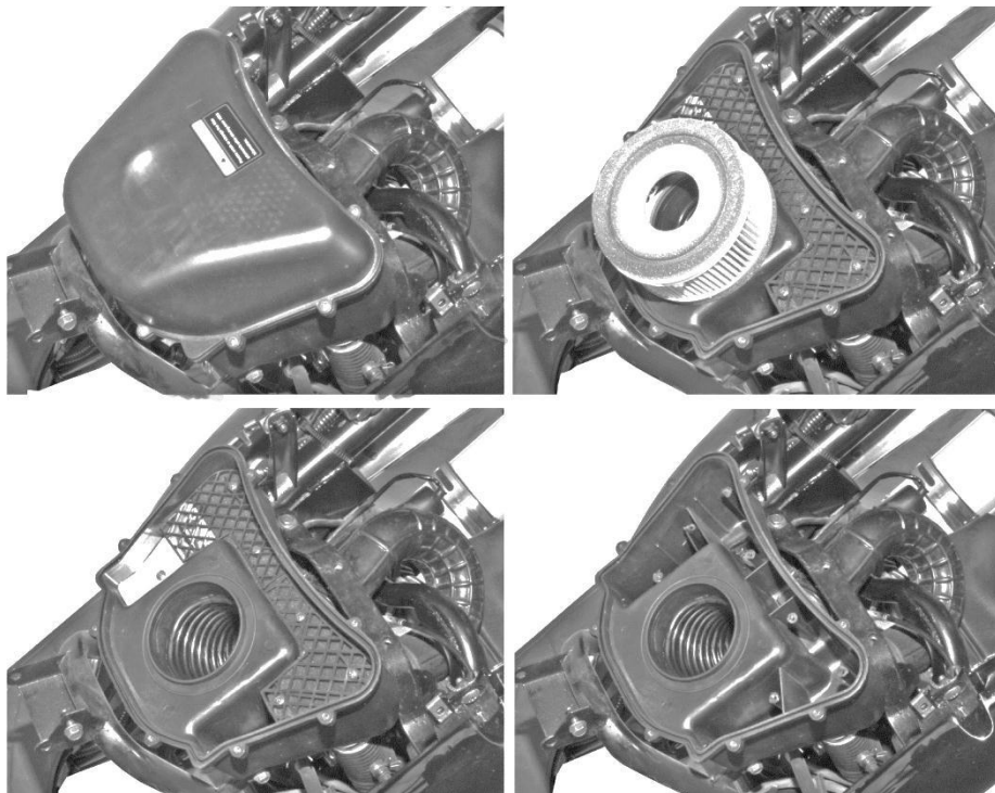
Рис. 6.6. Повітряний фільтр
