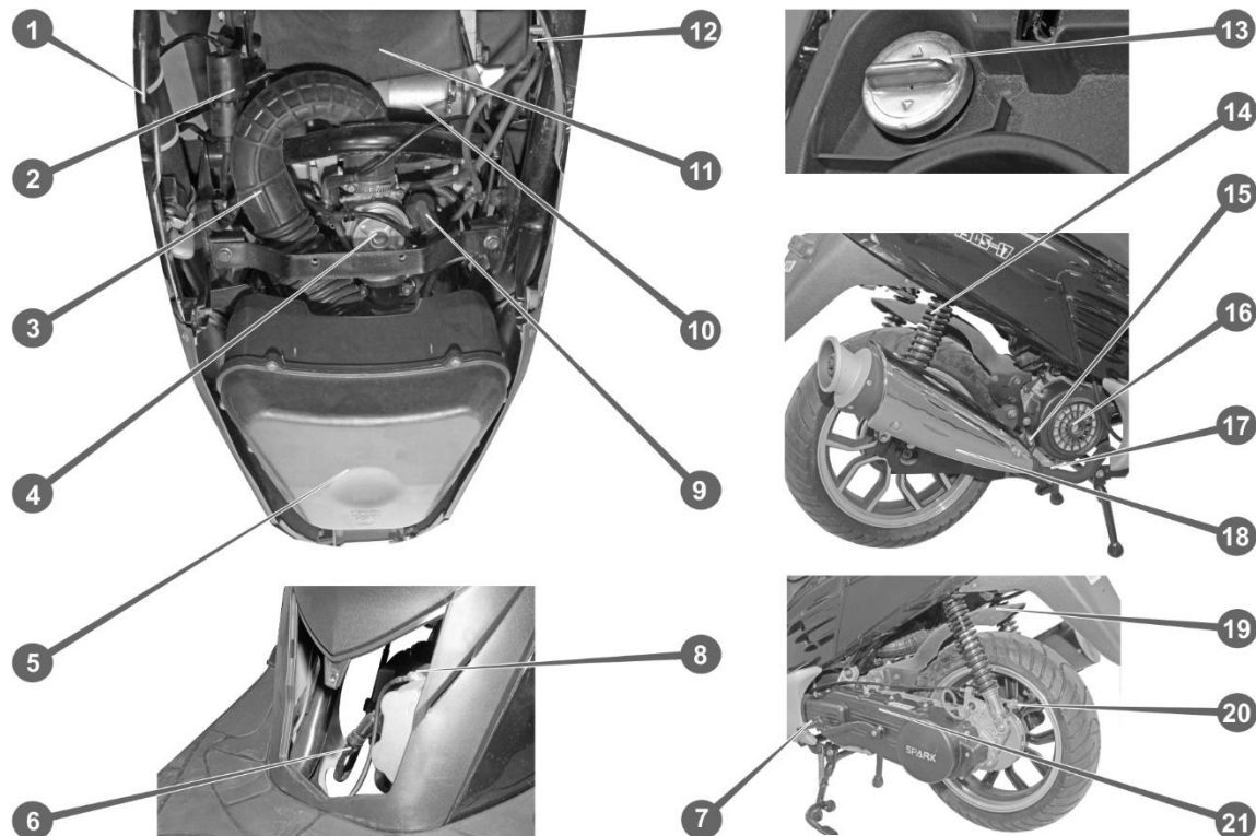
Рис. 3.3. Силовий агрегат
