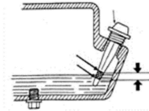
Рис. 6.1. Перевірка рівня мастила у двигуні Для перевірки рівня мастила необхідно пробку-щуп (див. рис. 6.2.). Вставити в заливну горловину, при цьому не закручуючи
