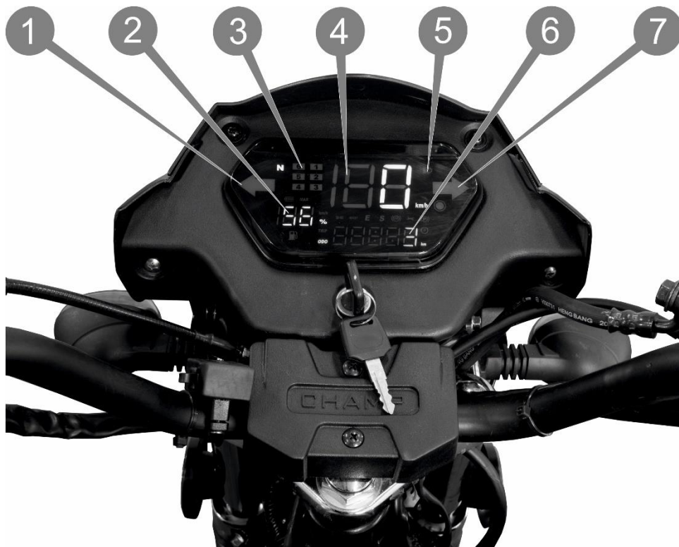
Рис. 3. Приладова панель
