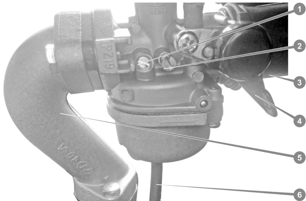
Рис. 7. Карбюратор
