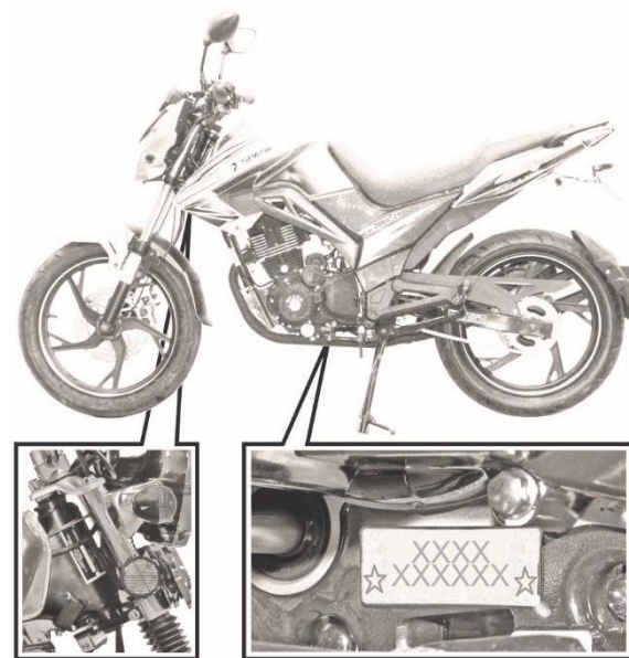
Рисунок 3.4. Розташування номера двигуна мотоцикла
