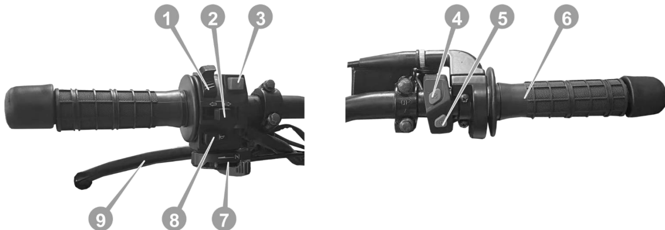
Рисунок 3.3. Блоки перемикачей.
