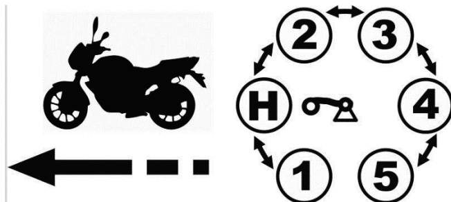
Рисунок 4.2. Схема перемикання передач
