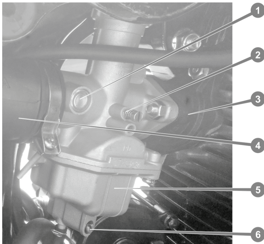
Рисунок 3.6.1. Карбюратор
