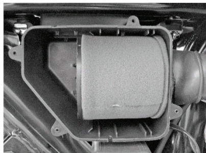
Рисунок 6.5. Повітряний фільтр і фільтрувальний елемент*
