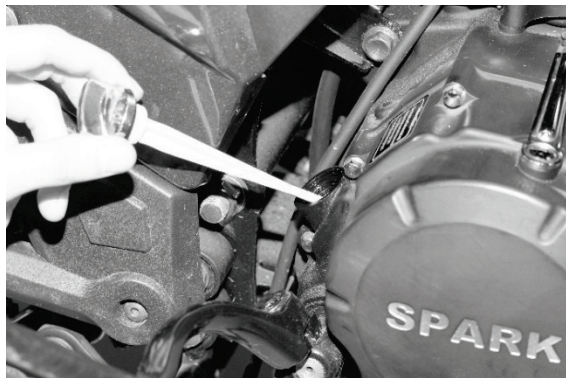
Рисунок 6.1. Пробка-щуп мастила картера двигуна
