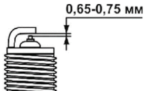
Рис. 6.4. Свічка запалювання, регулювання зазору.
