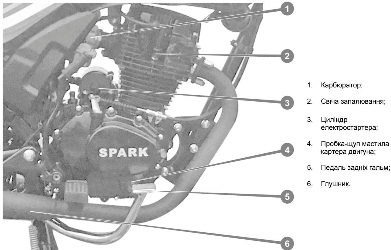
Рисунок 3.5. Вид двигуна праворуч
