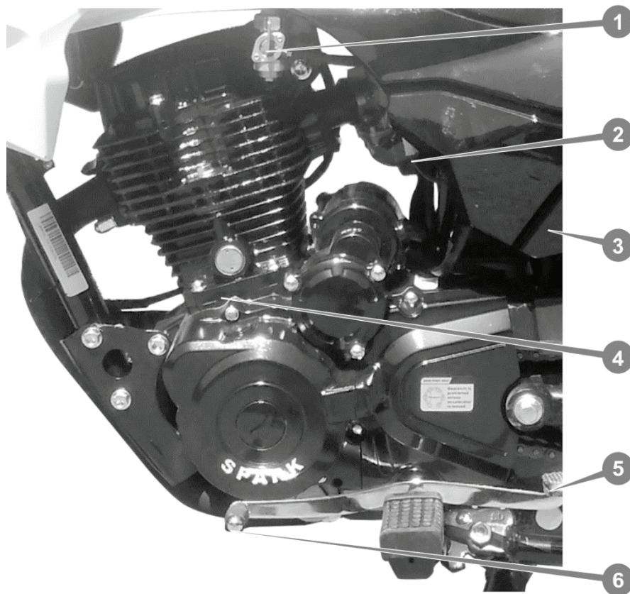
Рисунок 3.4. Вид двигуна ліворуч
