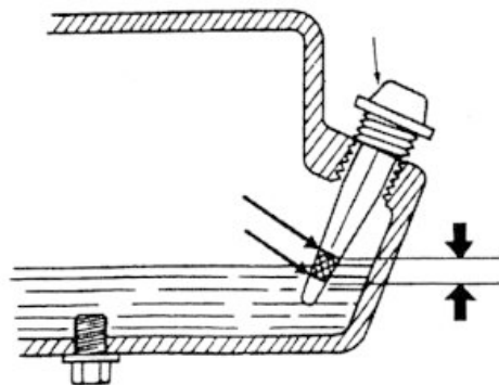
Рисунок 6.2. Перевірка рівня мастила у двигуні
