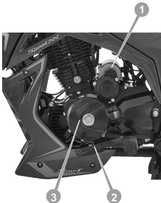
Рисунок 5. Вид двигуна ліворуч
