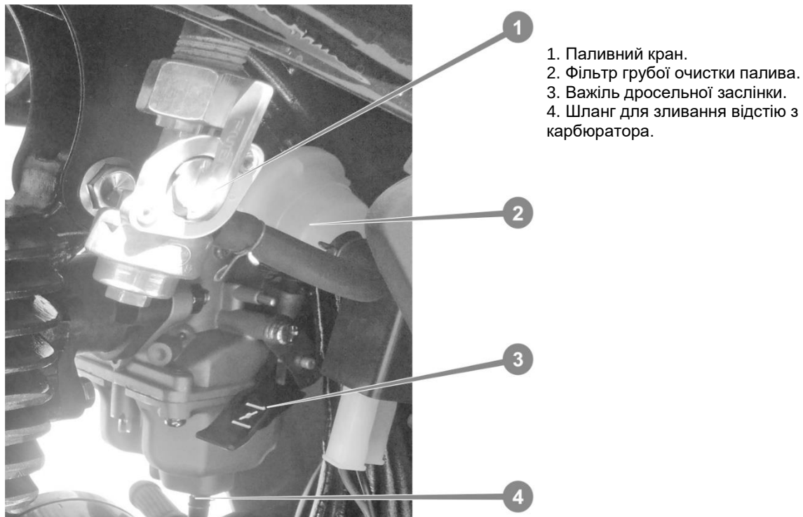
Рисунок 7.2. Карбюратор
