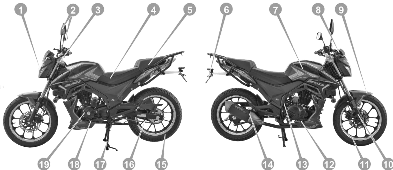
Рисунок 1. Основні вузли та агрегати
