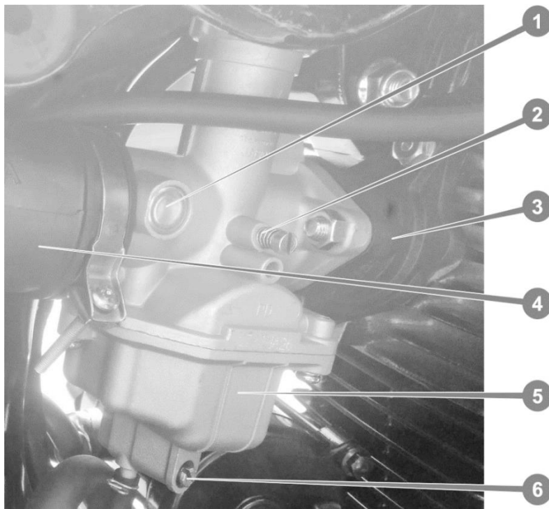
Рисунок 7.1. Карбюратор*
