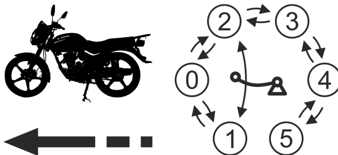
Рисунок 9. Схема перемикання передач
