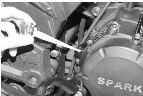
Рисунок 11. Пробка-щуп мастила картера двигуна
