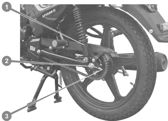
Рисунок 16. Ланцюгова передача і маятникова підвіска
