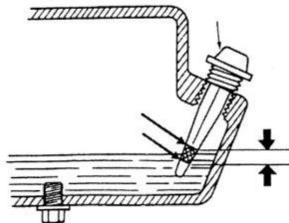
Рисунок 12. Перевірка рівня мастила у двигуні
