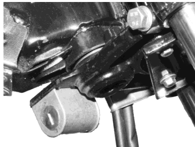
Рисунок 10. Замок блокування керма
