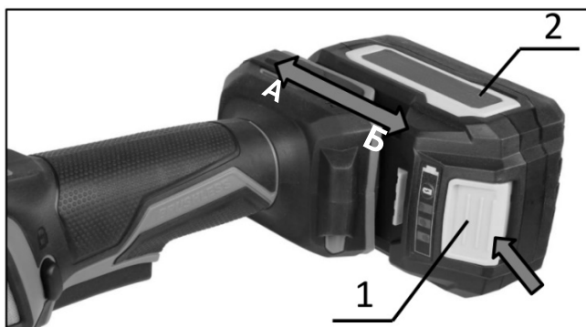
Рисунок 9. Схема встановлення (зняття) акумуляторної батареї.
