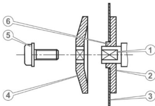
Рисунок 2. Встановлення циркулярного диска.
