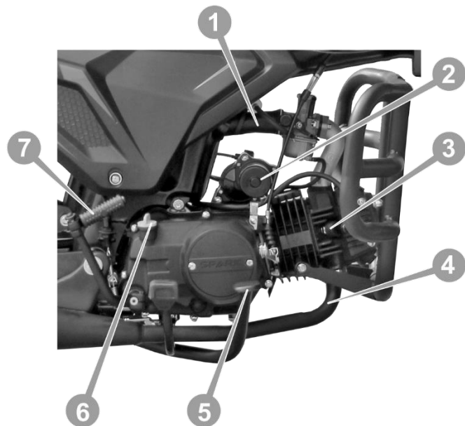
Рис. 5. Двигун, вид справа.
