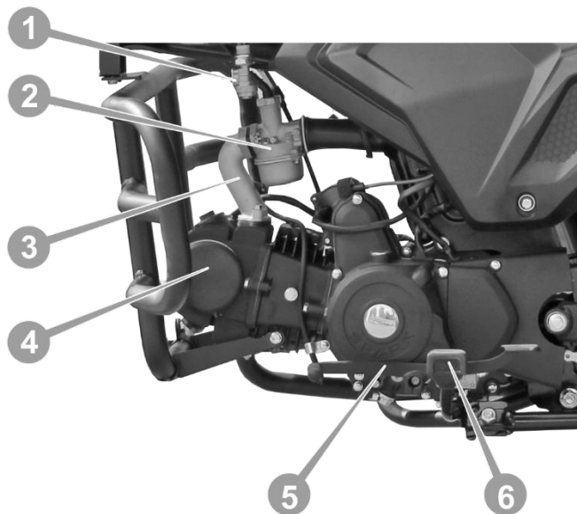
Рис. 4. Двигун, вид зліва.
