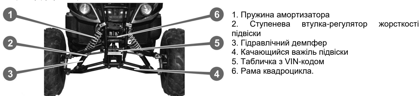
Рисунок 7.9. Передній міст
