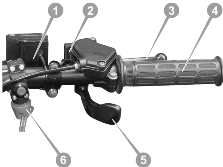
Рисунок 3.5. Блок перемикачів правий
