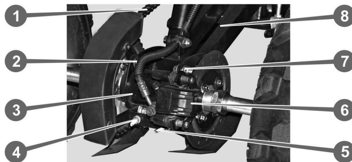
Рисунок 7.8. Механізм натягу ланцюга.
