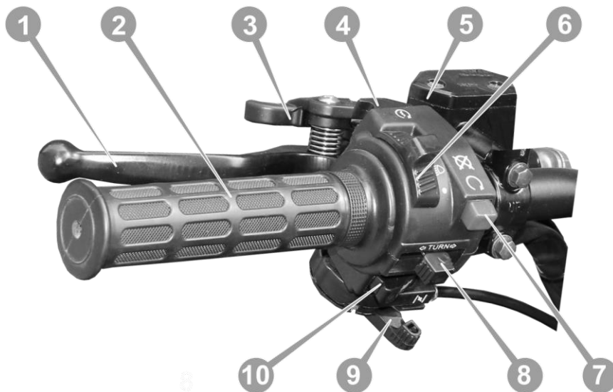
Рисунок 3.4. Блок перемикачів лівий
