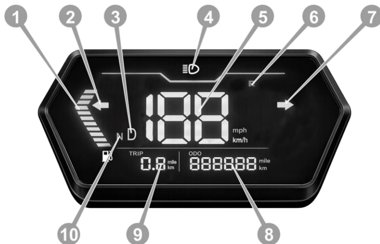
Рисунок 3.3. Панель приладів моделі SPARK APEX 125
