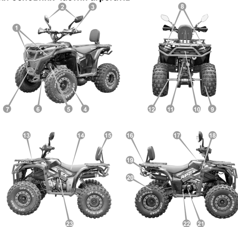
Рисунок 3.1. Розташування вузлів та агрегатів моделей SPARK APEX 125
