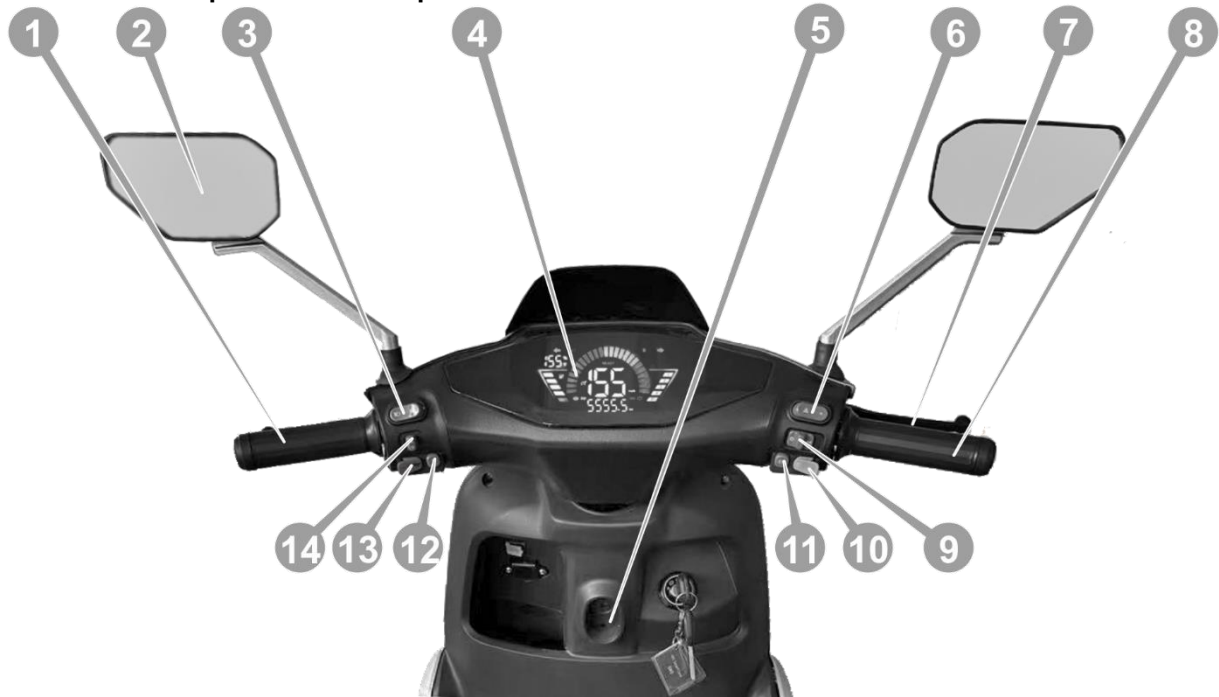
Рисунок 2.2. Кермо електроскутера, блоки керування на кермі
