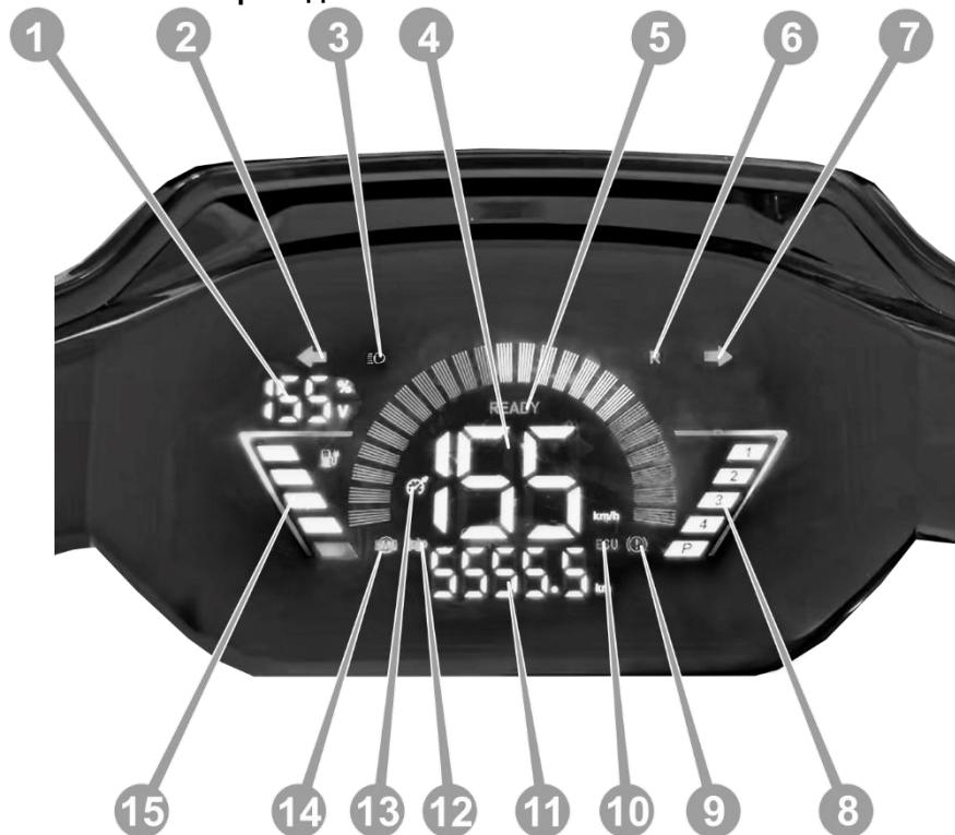
Рисунок 2.1. Панель приладів моделей електроскутера SP2000E-4
