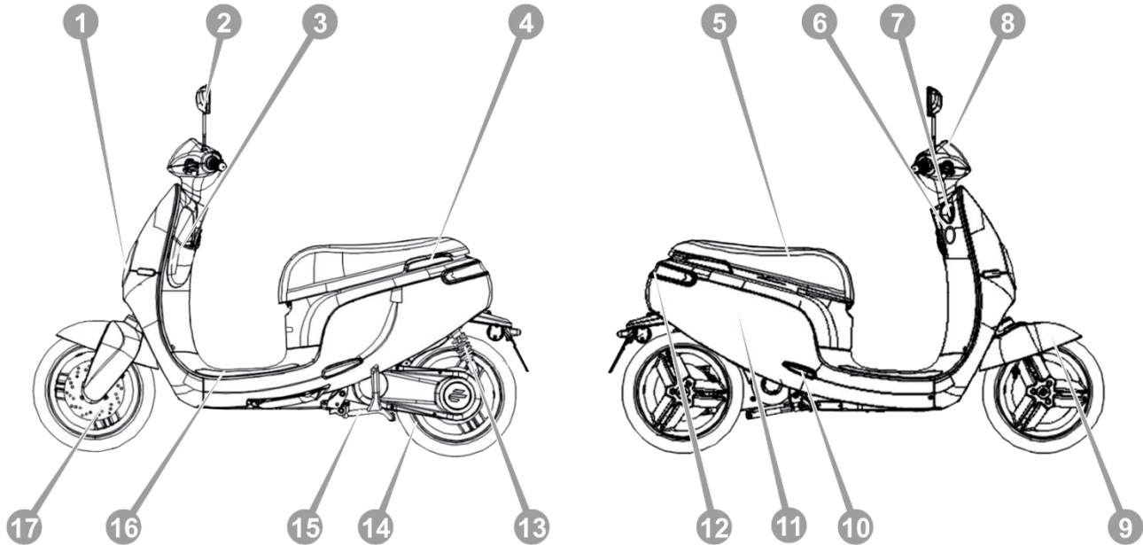
Рисунок 1.1. Загальний вигляд електроскутера.
