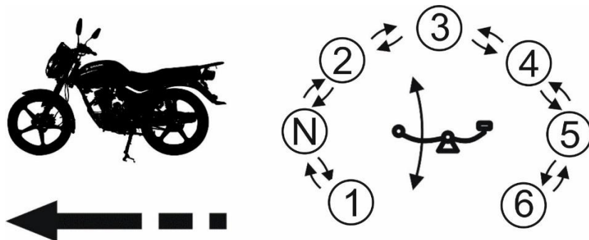
Рисунок 9. Схема перемикання передач
