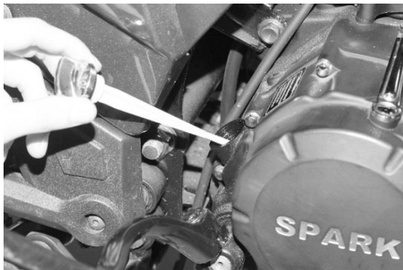
Рисунок 11. Пробка-щуп мастила картера двигуна
