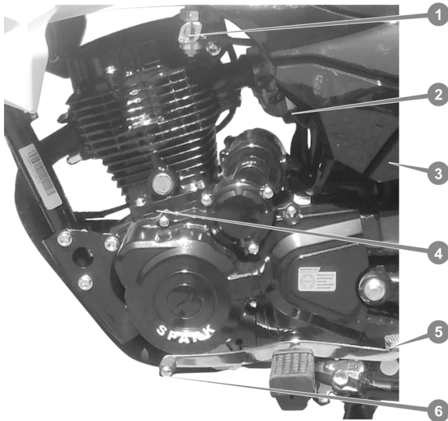
Рисунок 4. Вид двигуна ліворуч
