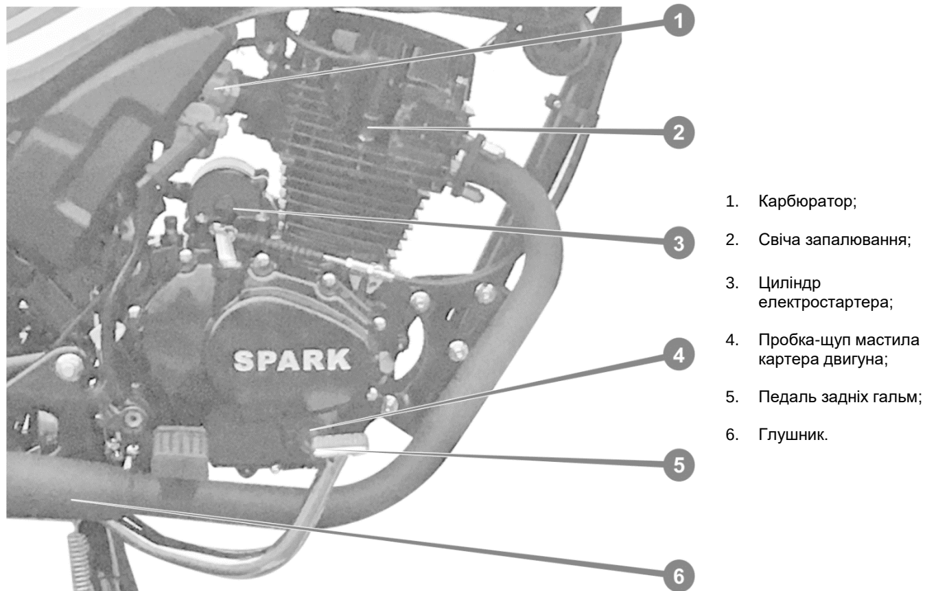
Рисунок 5. Вид двигуна праворуч
