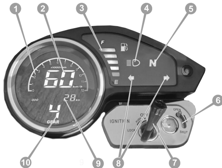
Рисунок 2. Приладова панель
