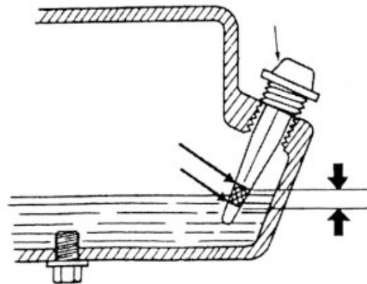
Рисунок 6.2. Положення пробки-щупа при вимірі рівня змащувального матеріалу
