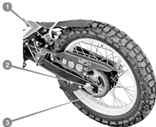
Рисунок 6.7. Ланцюгова передача і маятникова підвіска
