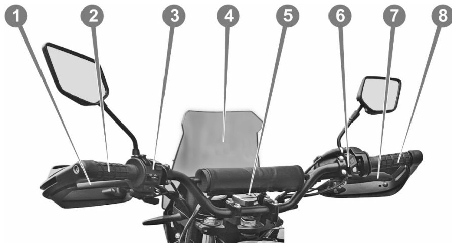
Рисунок 3.2. Загальний вид керма
