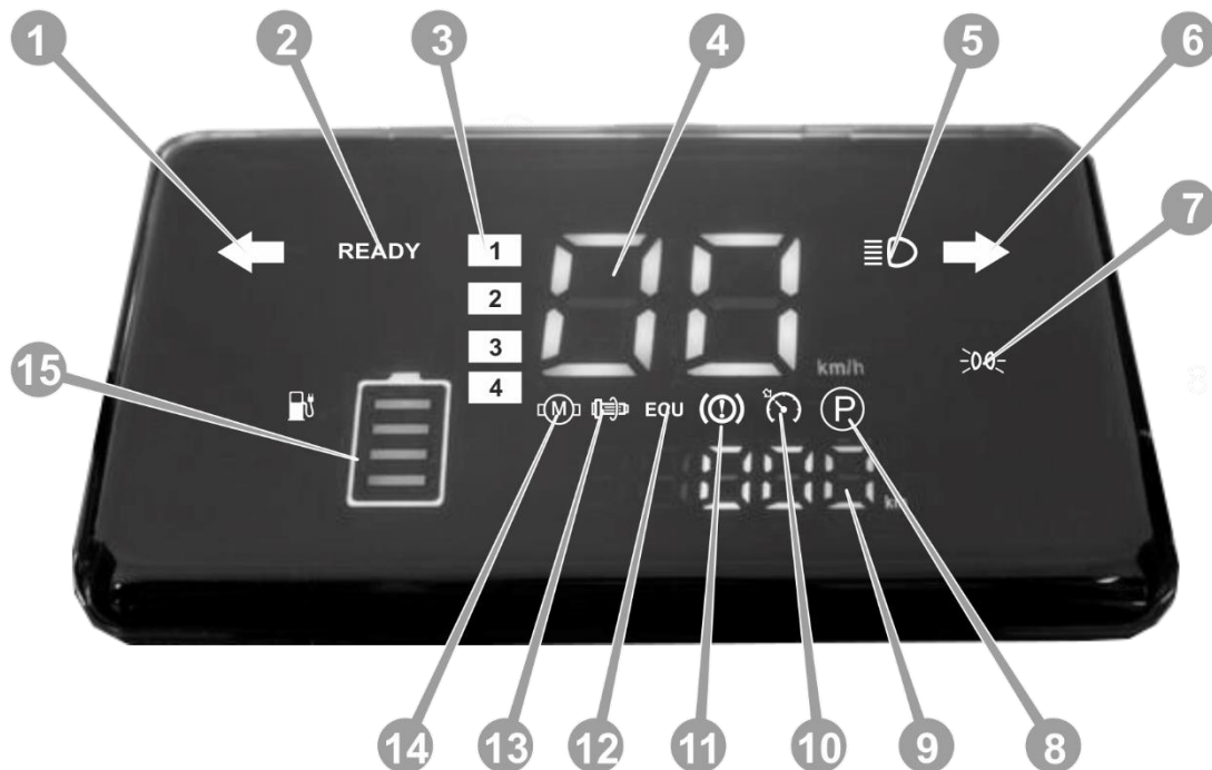
Рисунок 2.1. Панель приладів велосипеду з електромотором
