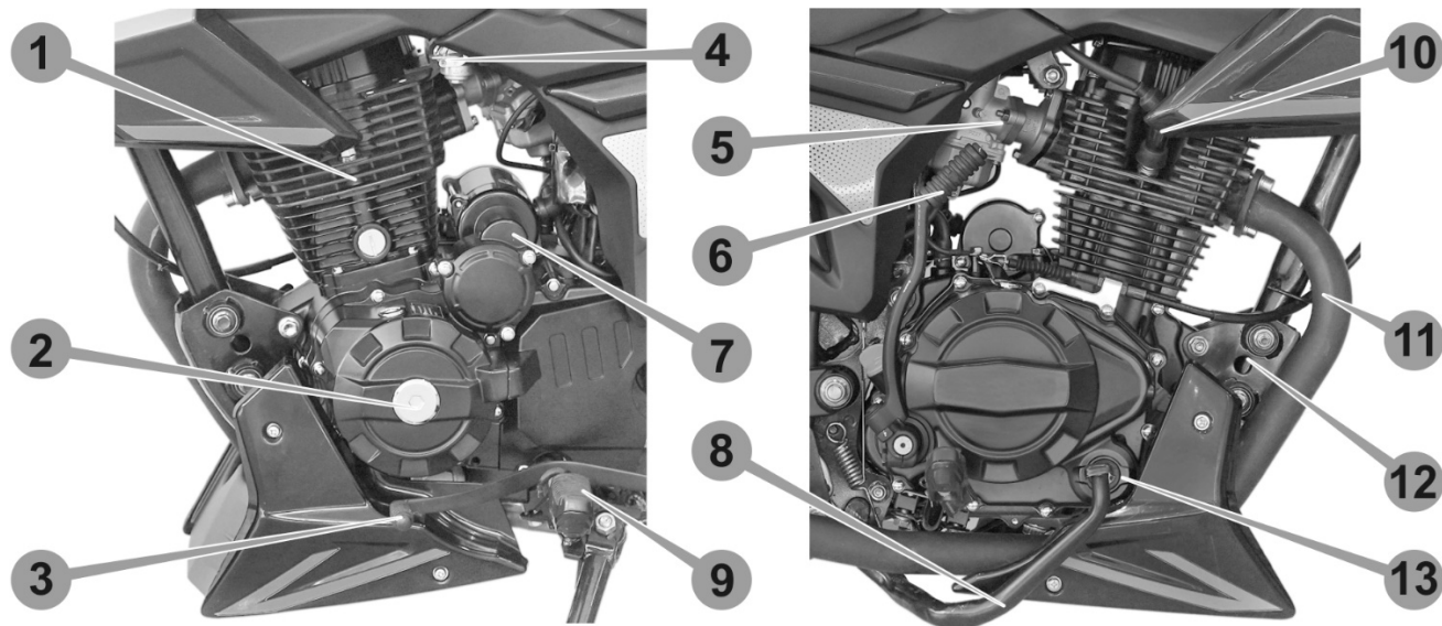
Рисунок 3.5. Двигун
