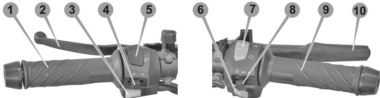
Рисунок 3.4. Блоки перемикачів.
