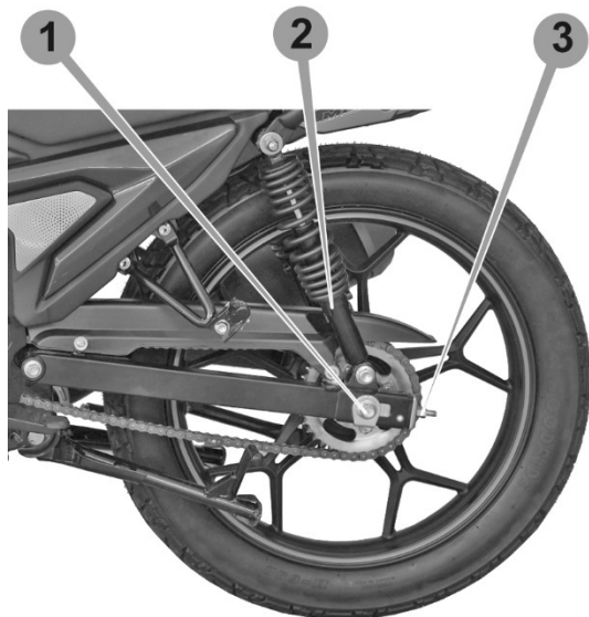
Рисунок 6.7. Регулювання натягу ланцюга і жорсткості амортизаторів
