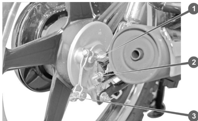
Рисунок 6.8. Заднє гальмо
