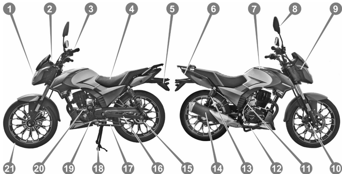
Рис. 3.1. Основні вузли й агрегати
