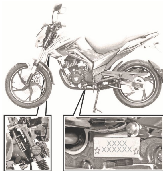
Рисунок 3.6. Розташування номера двигуна мотоцикла
