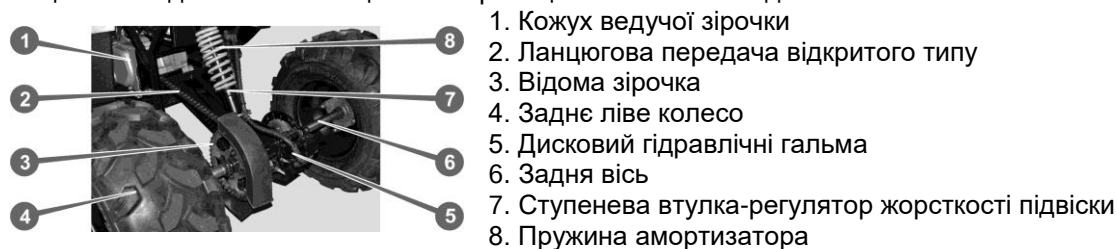
Рисунок 7.10. Задній міст
