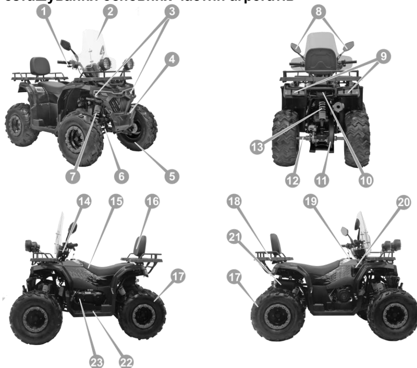
Рисунок 3.1.1 Розташування вузлів та агрегатів моделі SP200-10E (2026)
