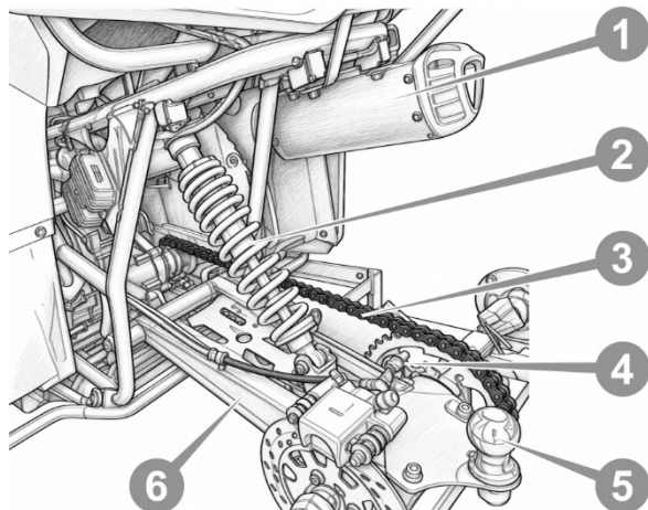
Рисунок 6.7. Механізм натягу ланцюга.
