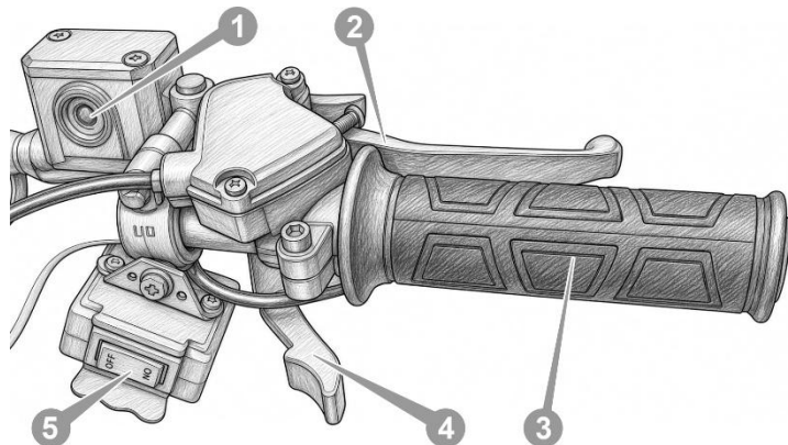
Рисунок 3.5. Блок перемикачів правий
