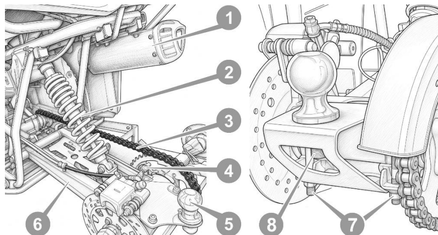
Рисунок 6.7. Механізм натягу ланцюга.
