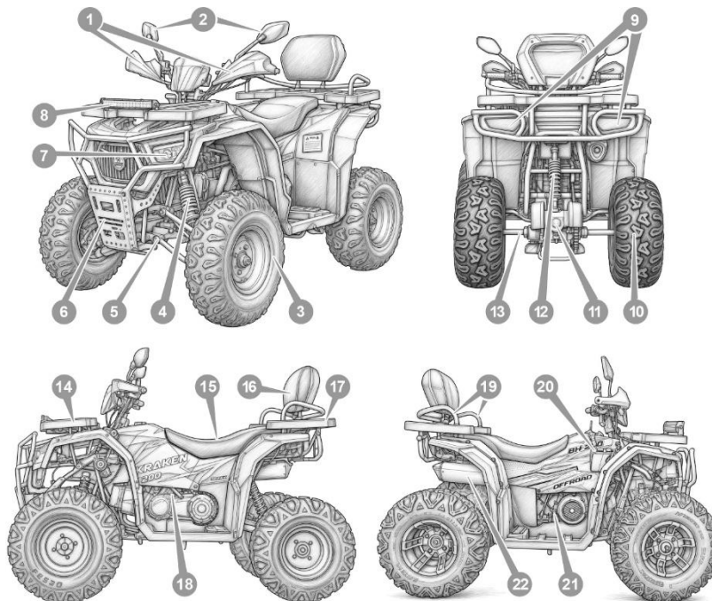
Рисунок 3.1. Розташування основних вузлів та агрегатів
