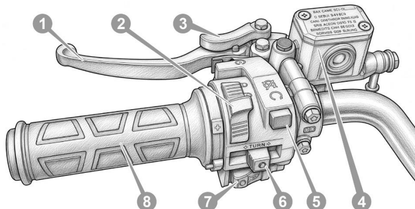
Рисунок 3.4. Блок перемикачів на кермі зліва
