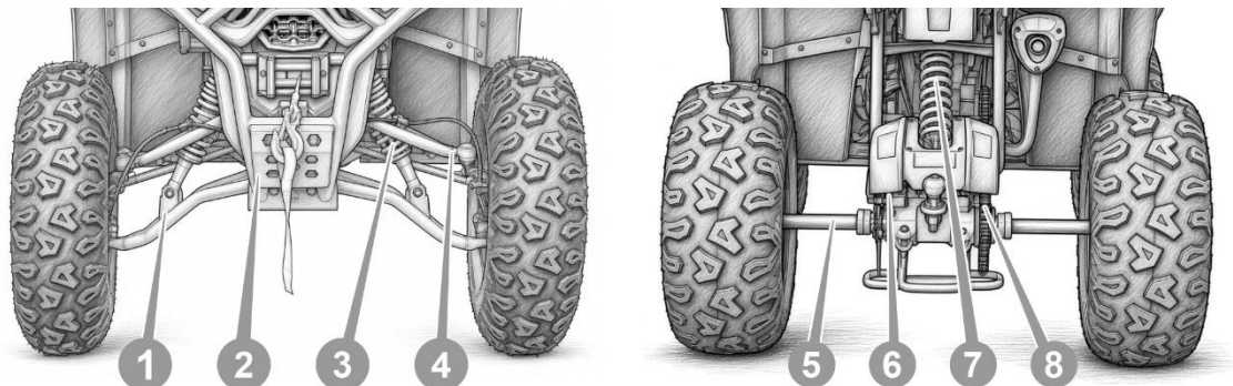
Рисунок 6.8. Ходова частина
