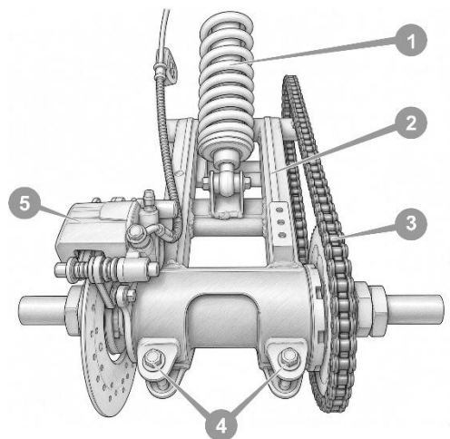
Рисунок 6.7. Механізм натягу ланцюга.
