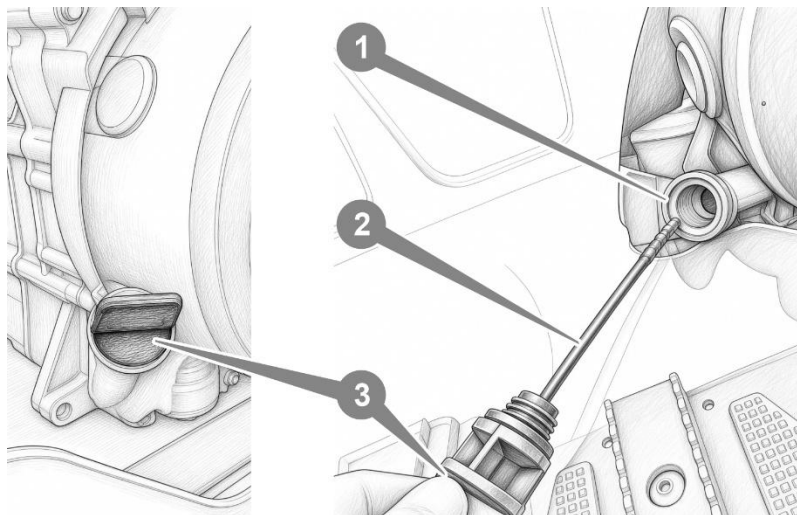
Рисунок 6.3. Перевірка рівня мастила в двигуні
