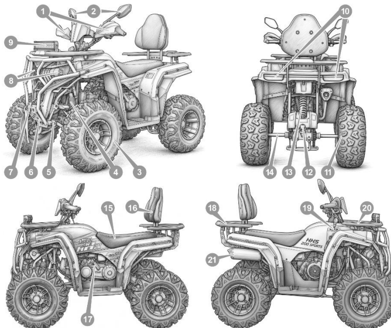
Рисунок 3.1. Розташування основних вузлів та агрегатів
