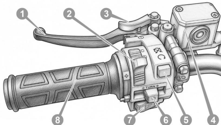
Рисунок 3.4. Блок перемикачів на кермі зліва
