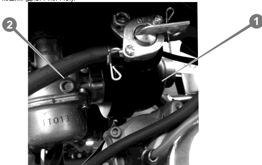
Рисунок 7.8. Повітряний фільтр, карбюратор
