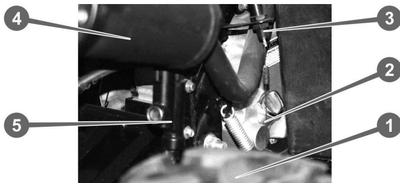
Рисунок 7.4. Заливна горловина картера двигуна
