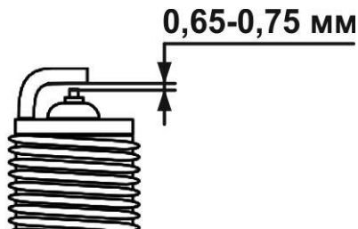
Рисунок 7.7. Свічка запалювання, регулювання зазору
