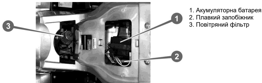
Рисунок 7.10. Вид зверху (Сидіння водія знято)
