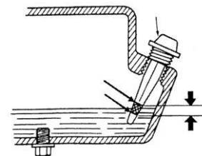
Рисунок 7.5. Перевірка рівня мастила в двигуні
