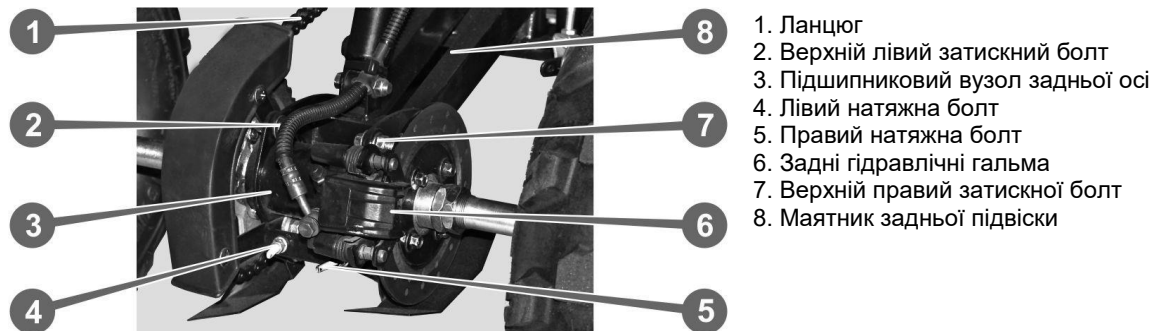
Рисунок 7.9. Механізм натягу ланцюга.
