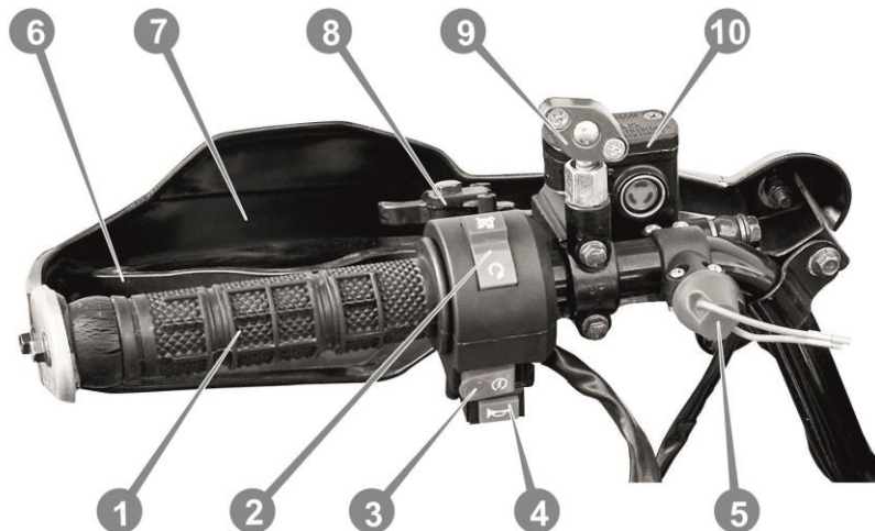
Рисунок 3.4. Блок перемикачів лівий
