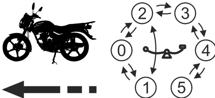
Рисунок 9. Схема перемикавання передач
