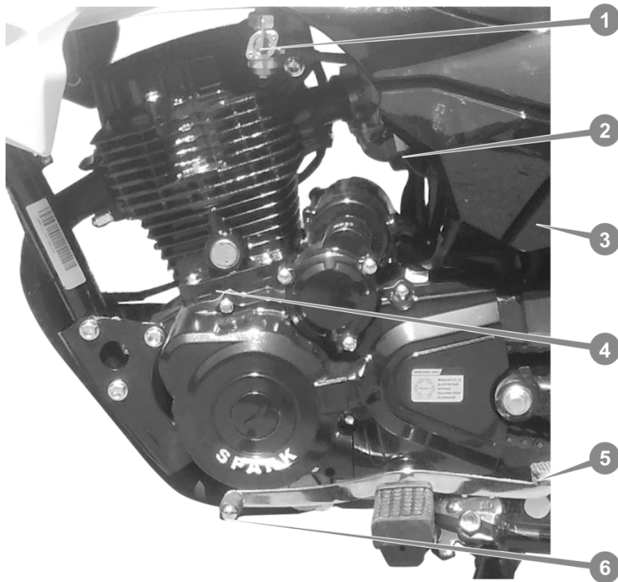
Рисунок 5. Вид двигуна ліворуч
