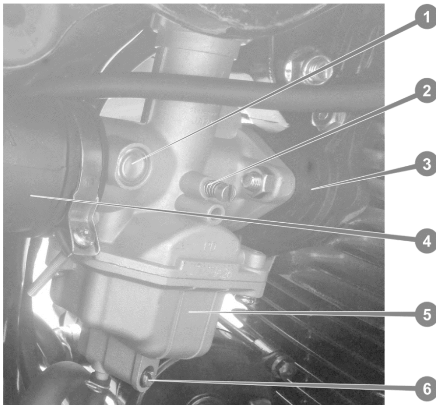
Рисунок 7.1. Карбюратор
