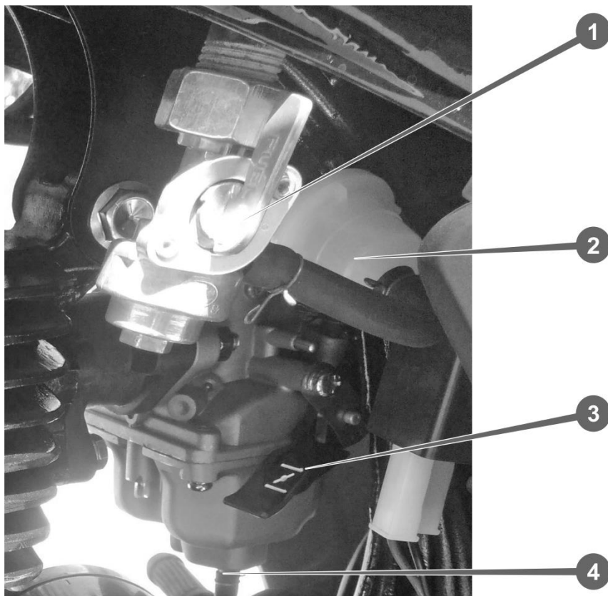
Рисунок 7.2. Карбюратор
