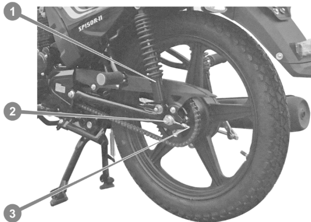
Рисунок 16. Ланцюгова передача і маятникова підвіска
