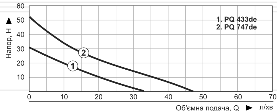
Графік продуктивності насосів серії PQ при 2850 об/хв
