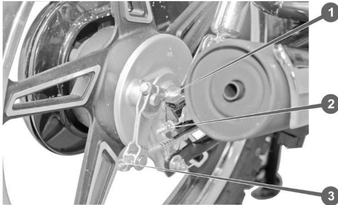
Рисунок 18. Заднє гальмо
