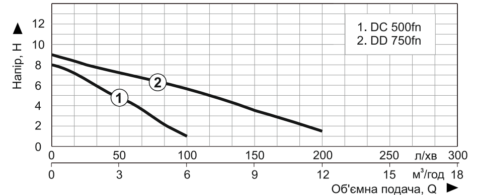
Продуктивність насосів при 2850 об/хв
