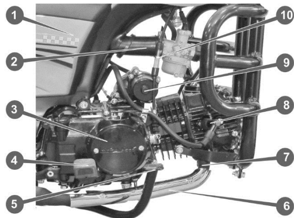
Рис. 3.6. Силовий агрегат, вид справа.
