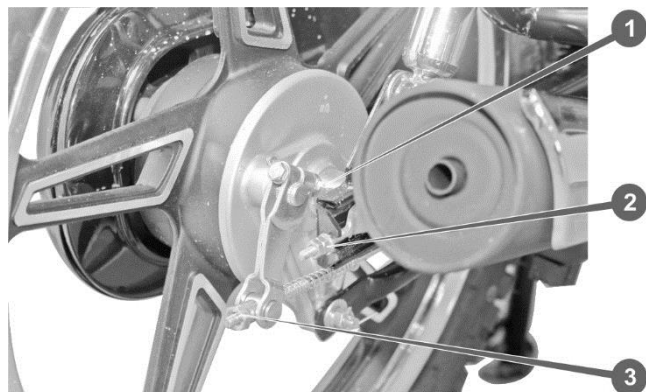
Рис. 6.2. Заднє гальмо
