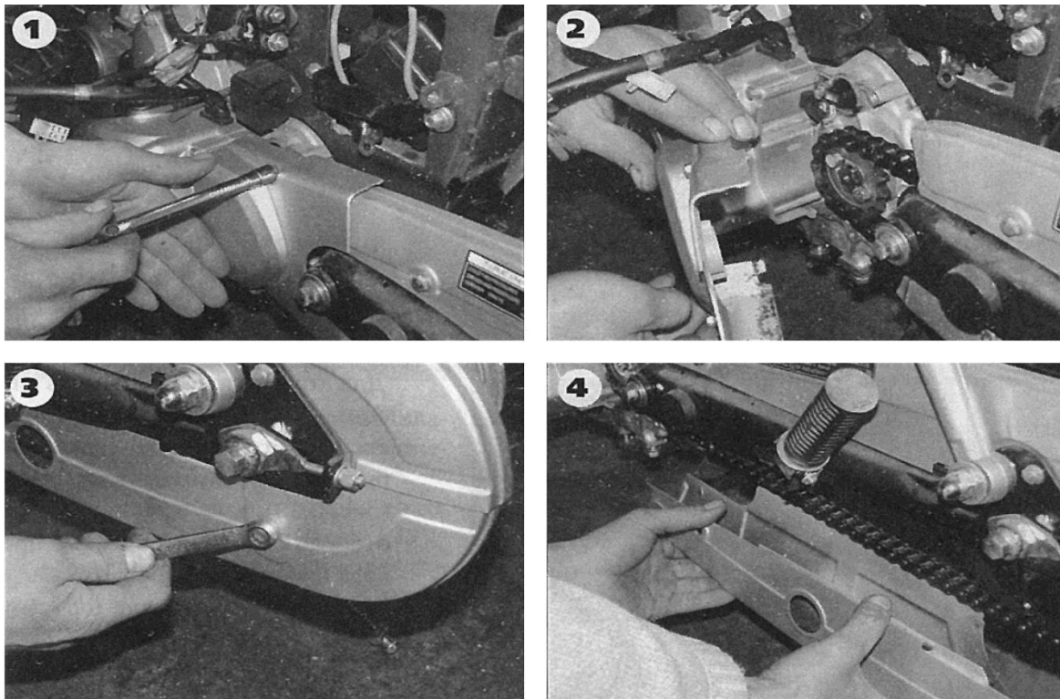
Рис. 5.8. Зняття кожуха ланцюгової передачі
