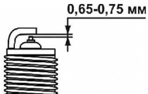
Рис. 5.4. Свічка запалювання, регулювання зазору.
