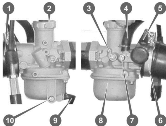
Рис. 5.6. Карбюратор
