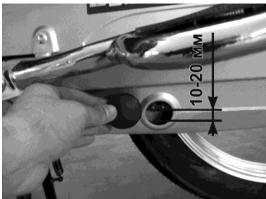
Рис. 5.9. Перевірка провисання ланцюга
