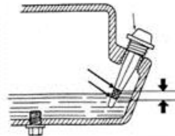
Рис. 5.2. Положення щупа при замірі рівня масла
