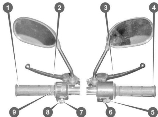
Рис. 3.4. Блоки перемикачів
