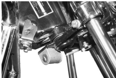
Рис. 4.3. Замок блокування керма
