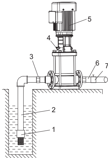
Коректний монтаж
