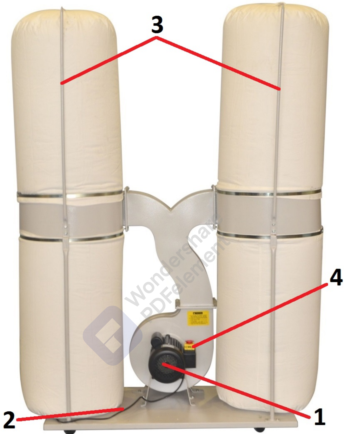
Мал. 1.2 Принципова будова верстата
