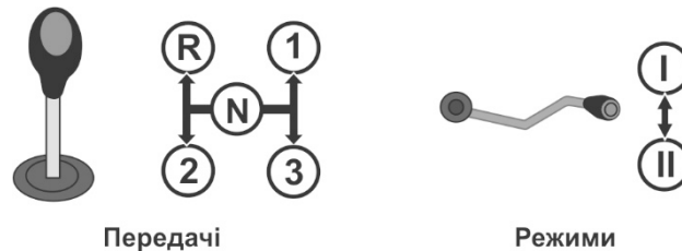
Рисунок 3.10. Перемикання передач і режимів трактора
