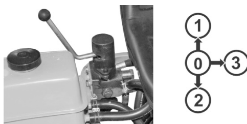
Рисунок 3.5.1. Положення важеля гідророзподільника
