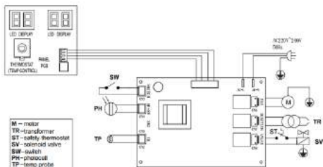
Wiring Diagram 90-082:
