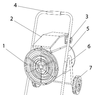
Рисунок 4. Модель «TCEF-30/3480»
