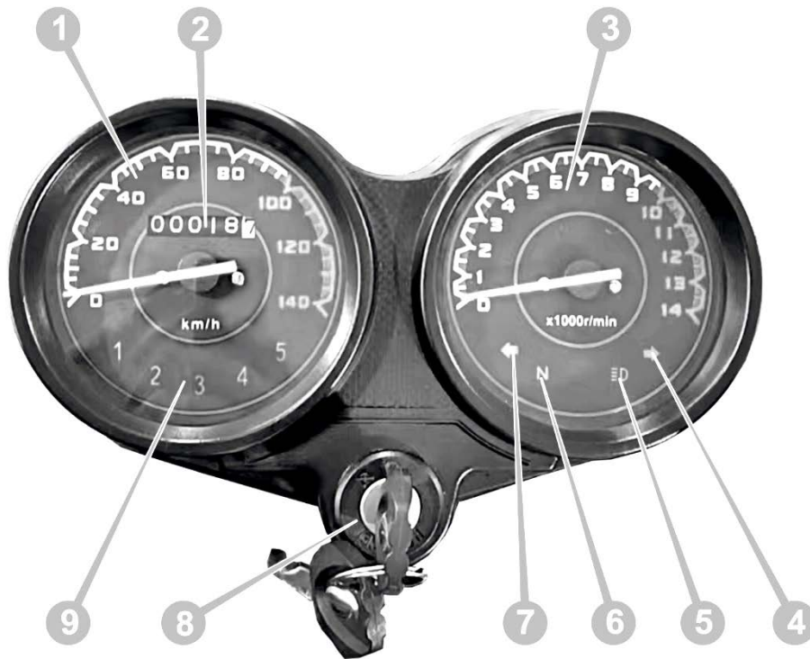
Рисунок 3. Панель приладів*
