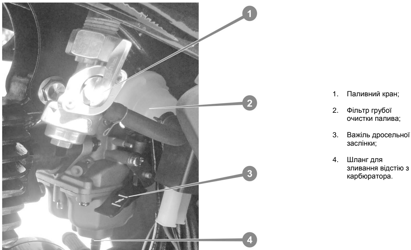
Рисунок 7.2. Карбюратор
