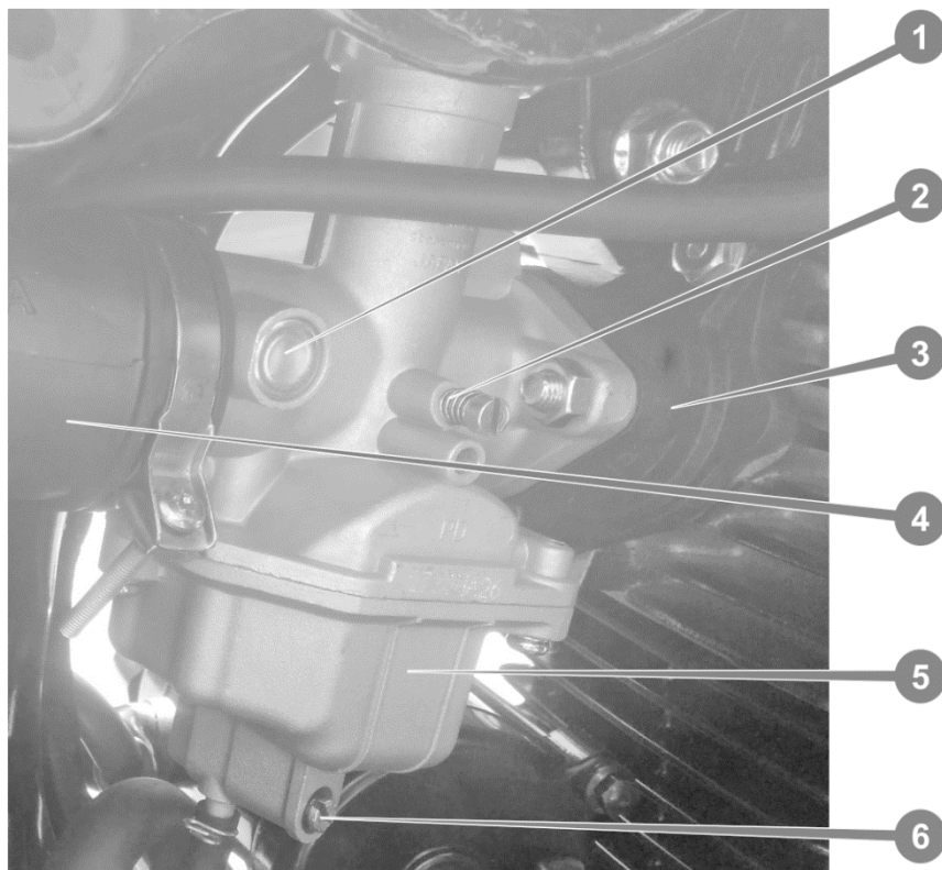
Рисунок 7.1. Карбюратор
