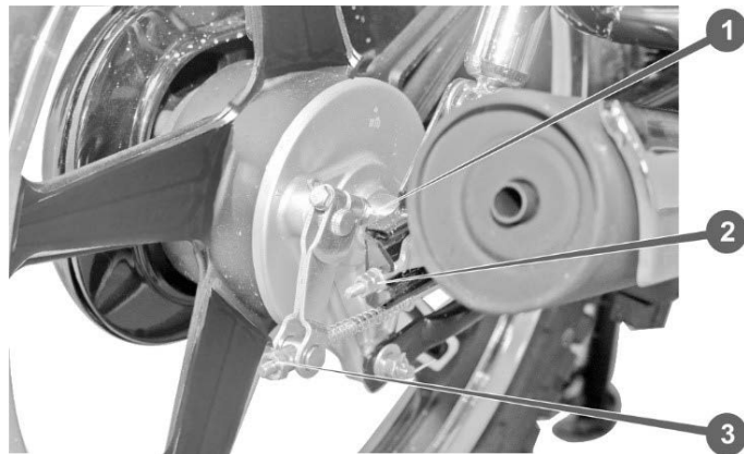
Рисунок 18. Заднє гальмо
