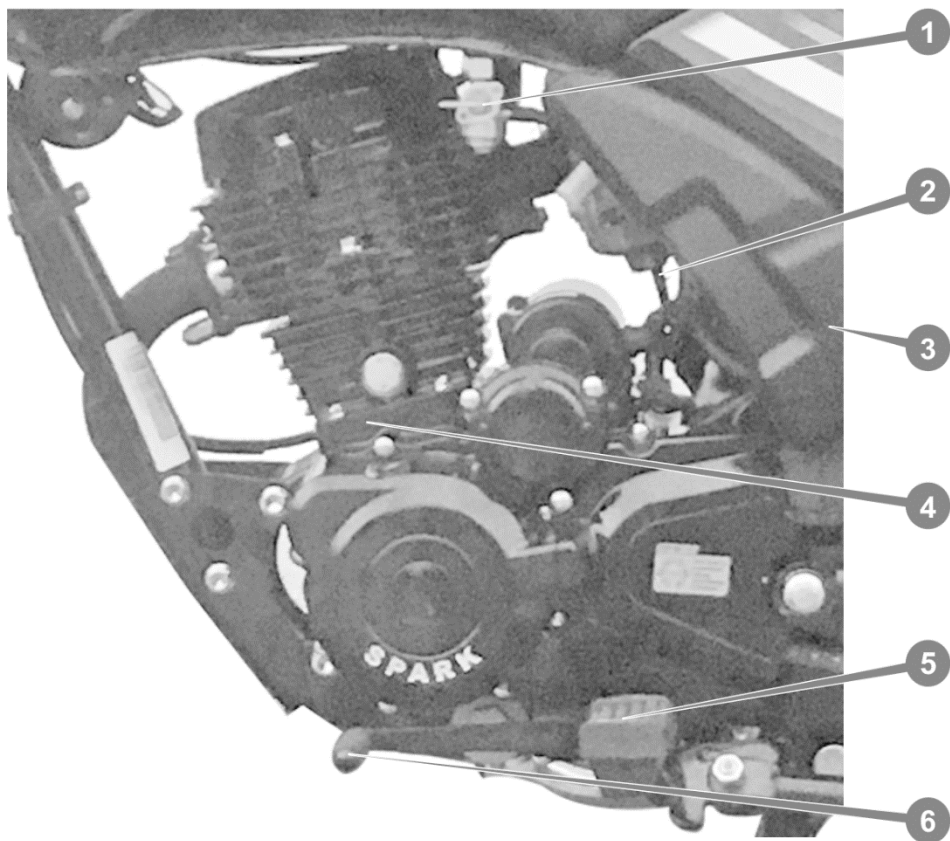
Рисунок 5. Вид двигуна ліворуч
