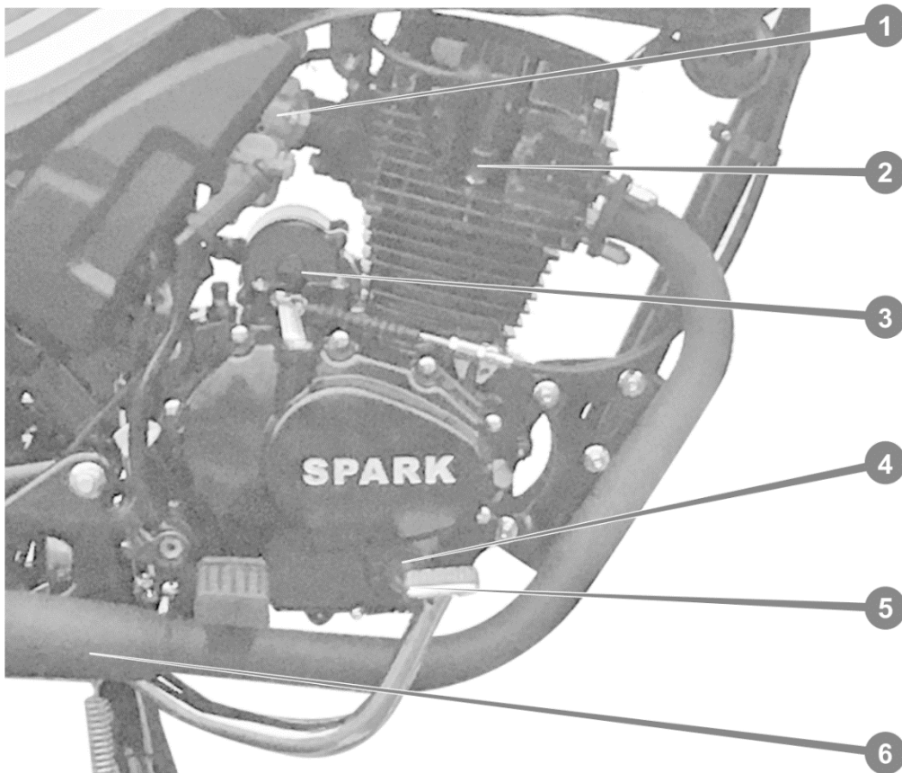
Рисунок 6. Вид двигуна праворуч
