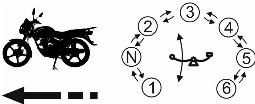
Рисунок 4.2. Схема перемикання передач
