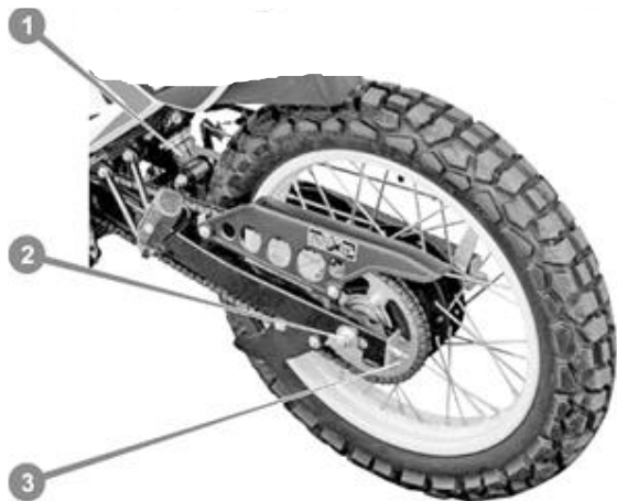
Рисунок 6.6. Ланцюгова передача і маятнікова підвіска
