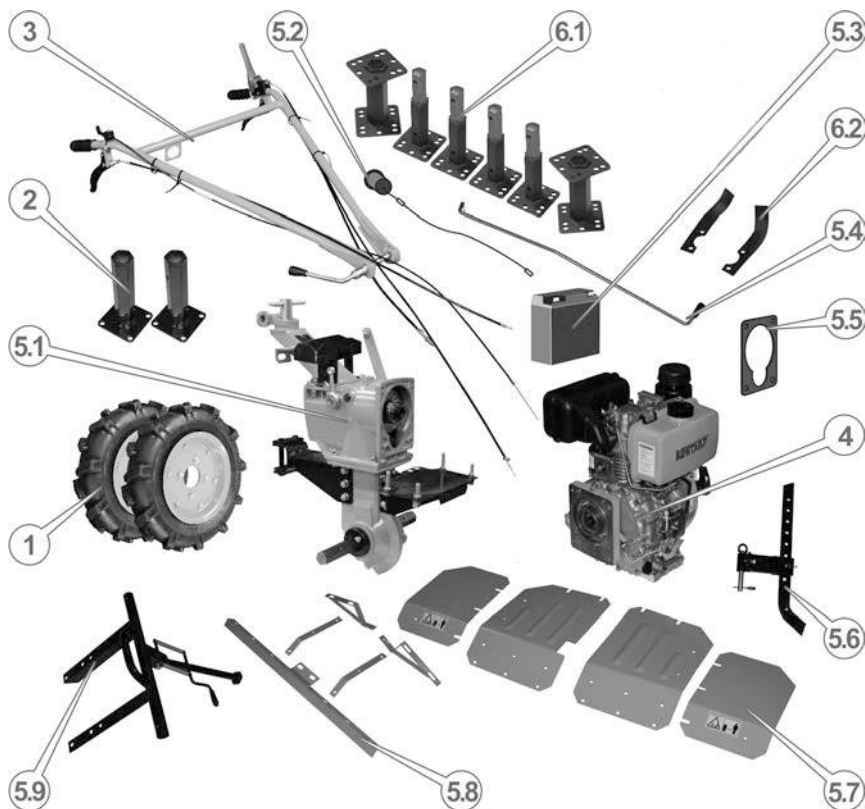
Рисунок 2 – Комплектація розширена
