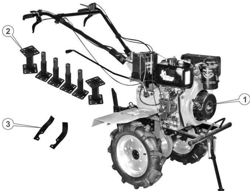
Рисунок 1 – Комплектація
