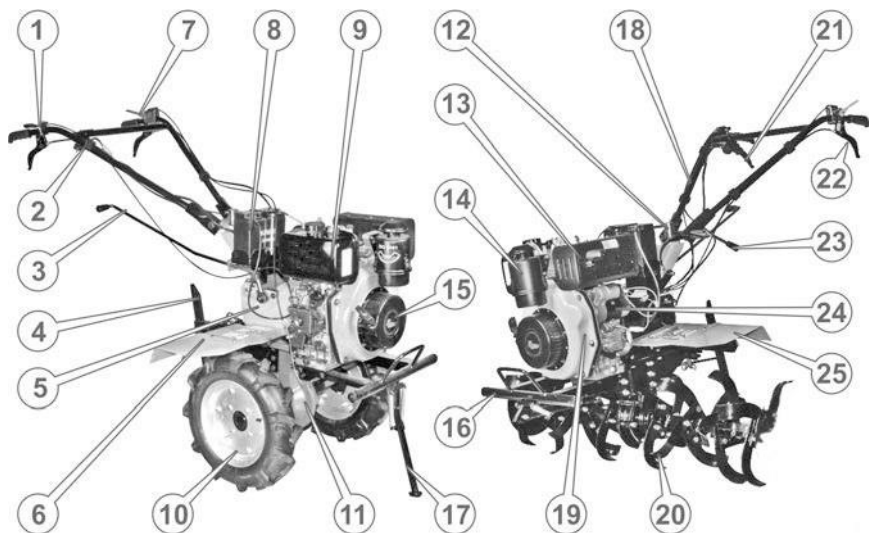
Рисунок 3 – Елементи мотоблока
