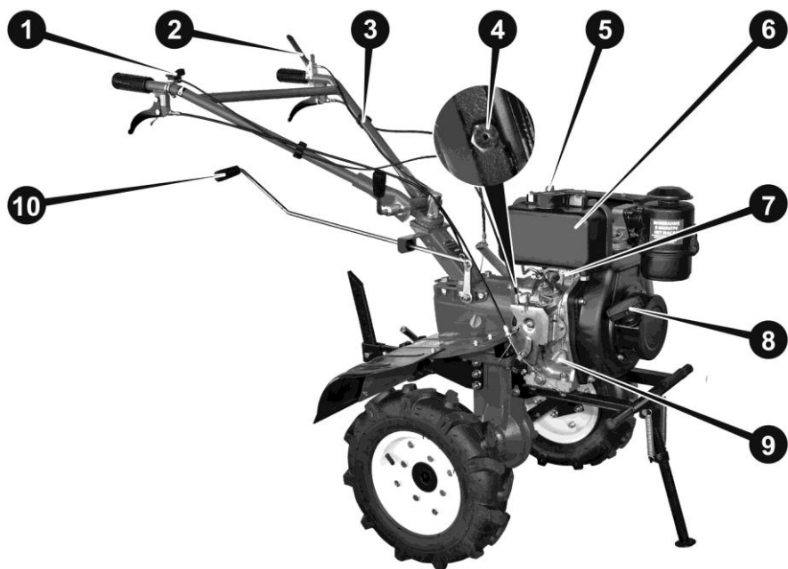
Рисунок 19 – Елементи регулювання
