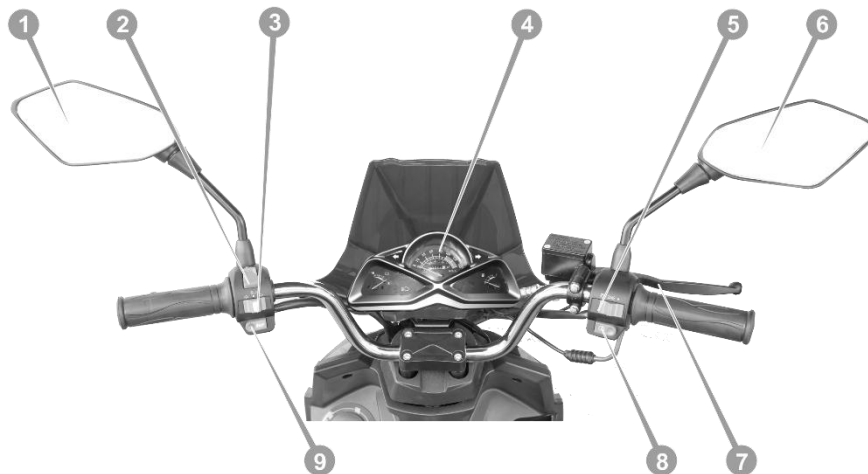
Рисунок 3.2.1. Органи керування
