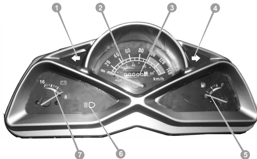
Рис.3.2.2. Панель приладів
