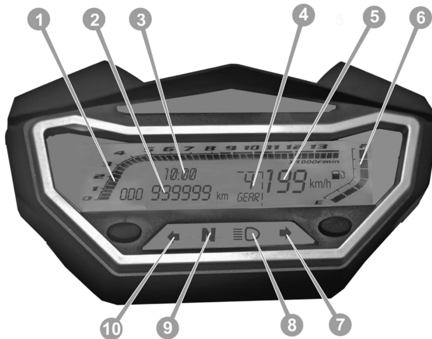
Рисунок 3.2. Приладова панель
