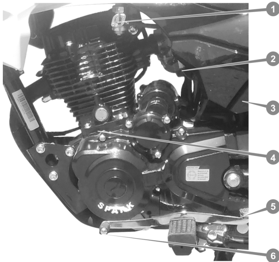
Рисунок 3.4. Вид двигуна ліворуч
