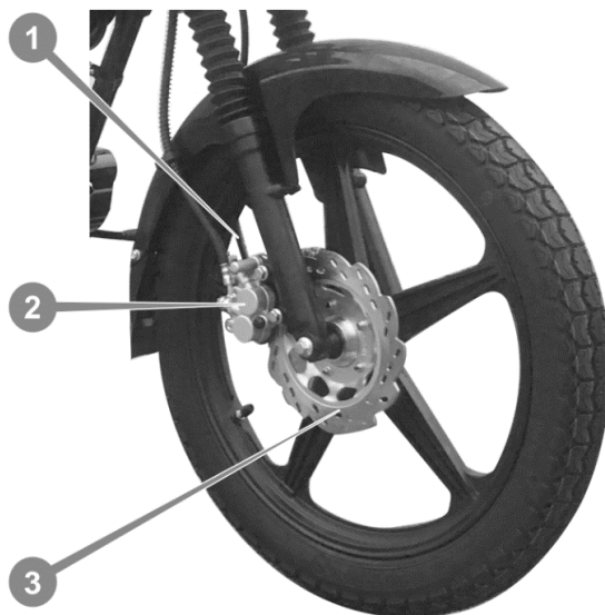
Рисунок 17. Переднє гальмо
