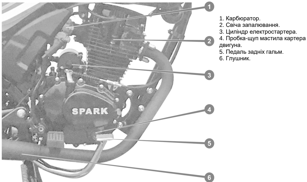
Рисунок 6. Вид двигуна праворуч
