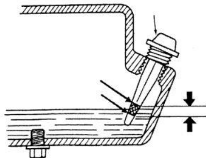
Рисунок 12. Перевірка рівня мастила у двигуні
