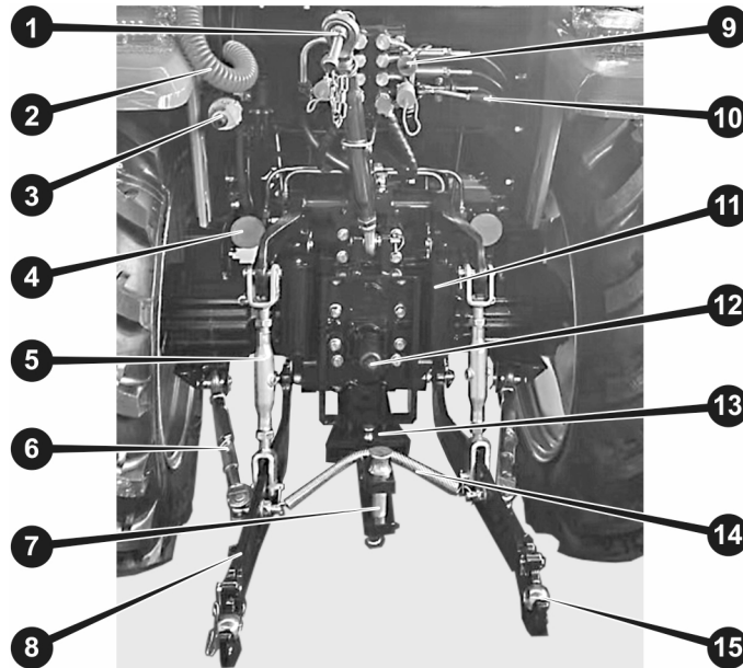
Рисунок 3.5. Триточкова гідронавісна система і вал відбору потужності
