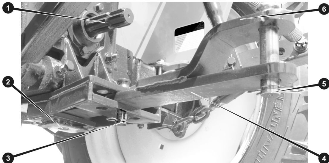
Рисунок 5.1. Тягово-зчипний пристрій
