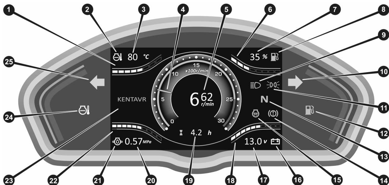
Рисунок 3.6. Панель приладів
