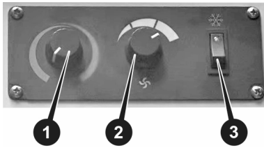
Рисунок 5.5. Панель керування кондиціонером
