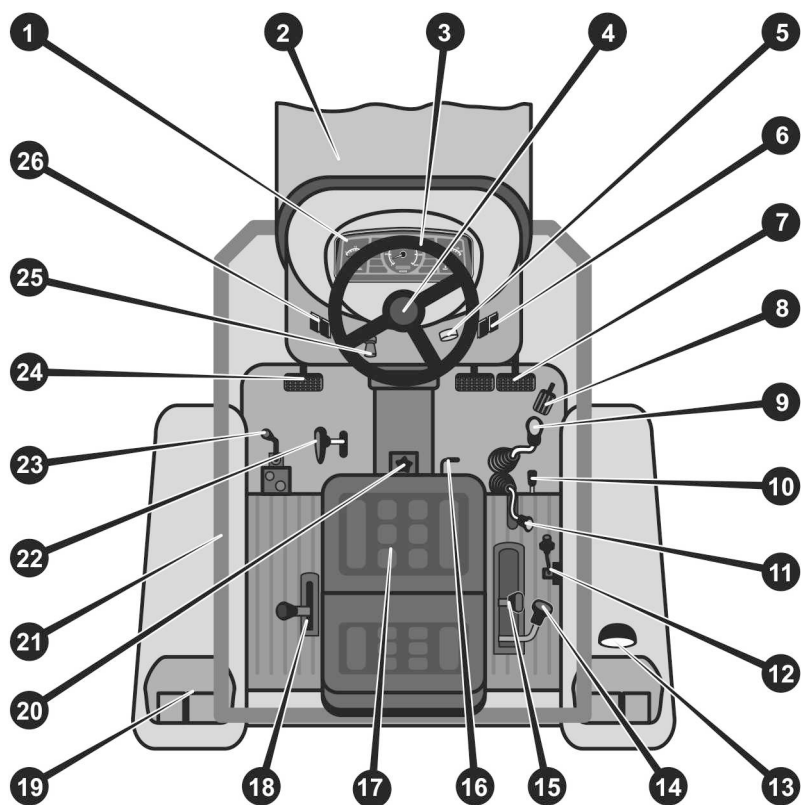
Рисунок 3.2. Схема розташування органів управління трактора KENTAVR 504
