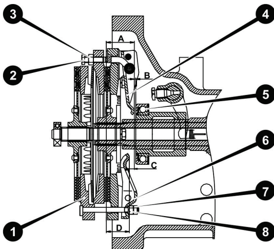
Рисунок 10.4. Муфта зчеплення дводискова
