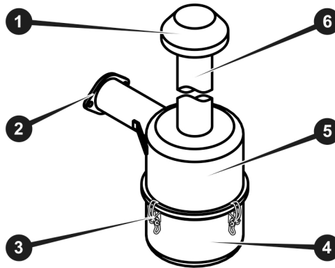
Рисунок 10.1. Повітряний фільтр
