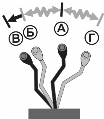
Рисунок 6.8 Положення важеля управління підйомником триточкової навісної системи
