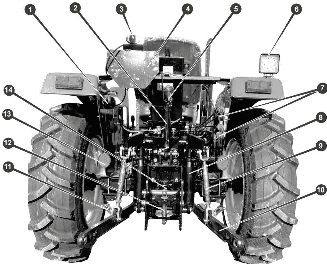
Рисунок 4.3. Триточкова гідронавісна система з двоходовим гідропідйомником
