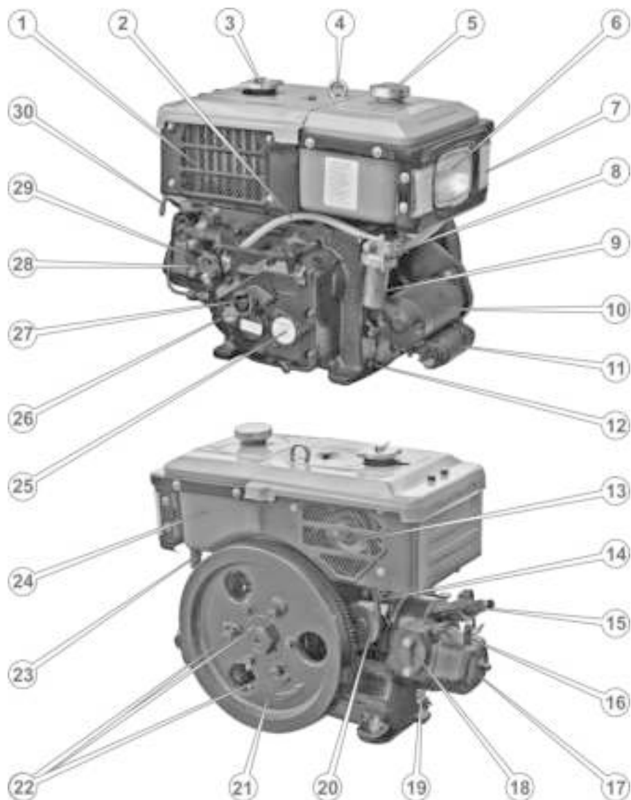
Рисунок 3. – Органи двигуна 180
