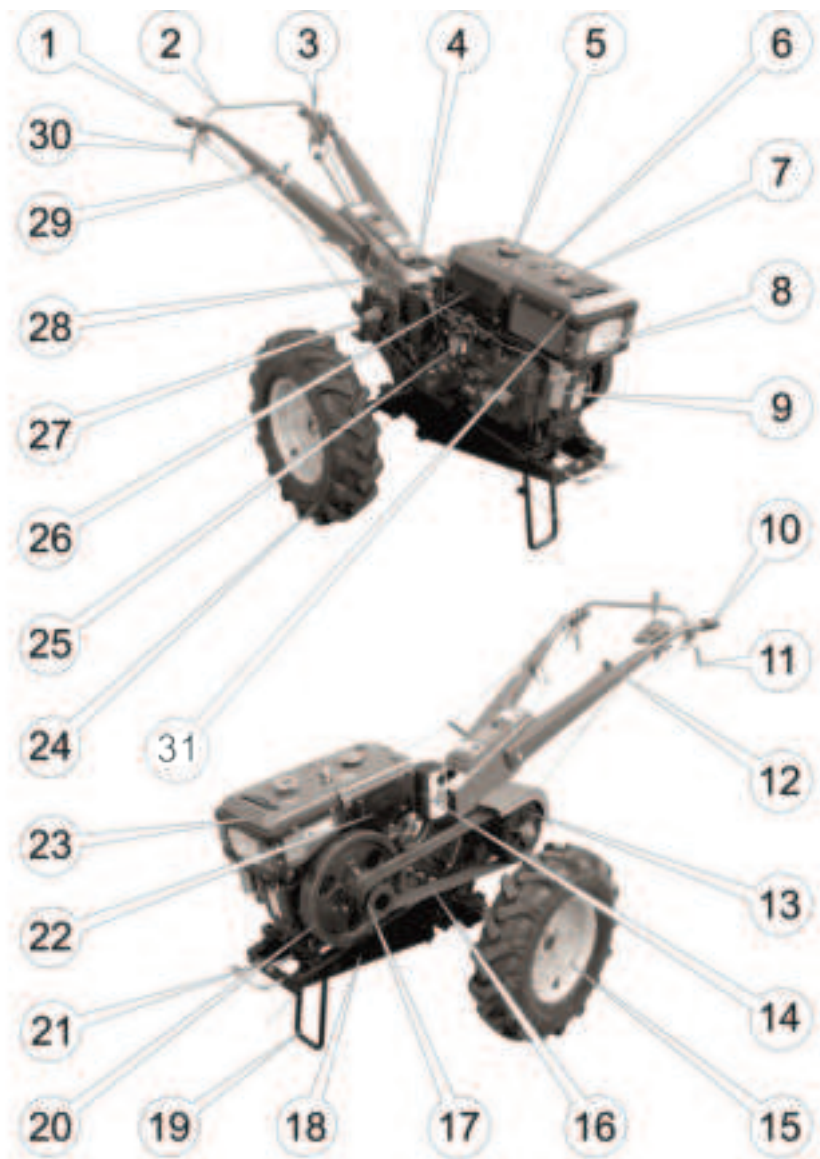
Рисунок 1. – Органи мотоблока МБ1080Д-10
