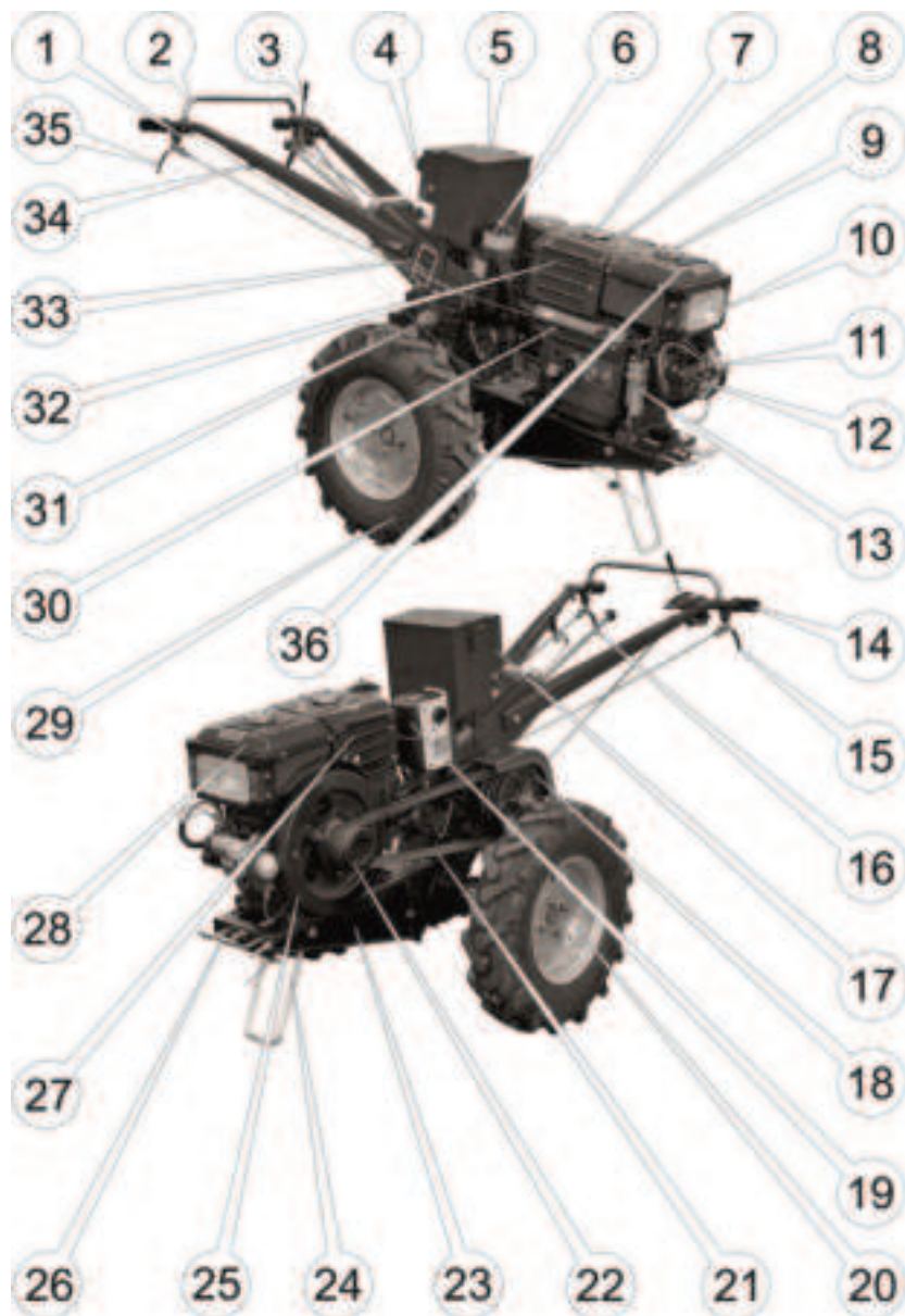
Рисунок 7. – Органи мотоблока МБ1012ДЕ-10
