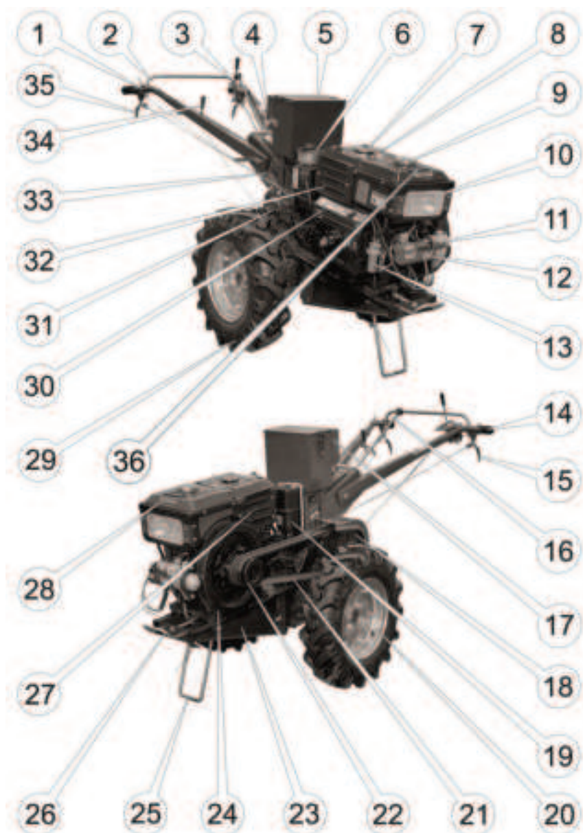
Рисунок. – 4. Органи мотоблока МБ1010ДЕ-10
