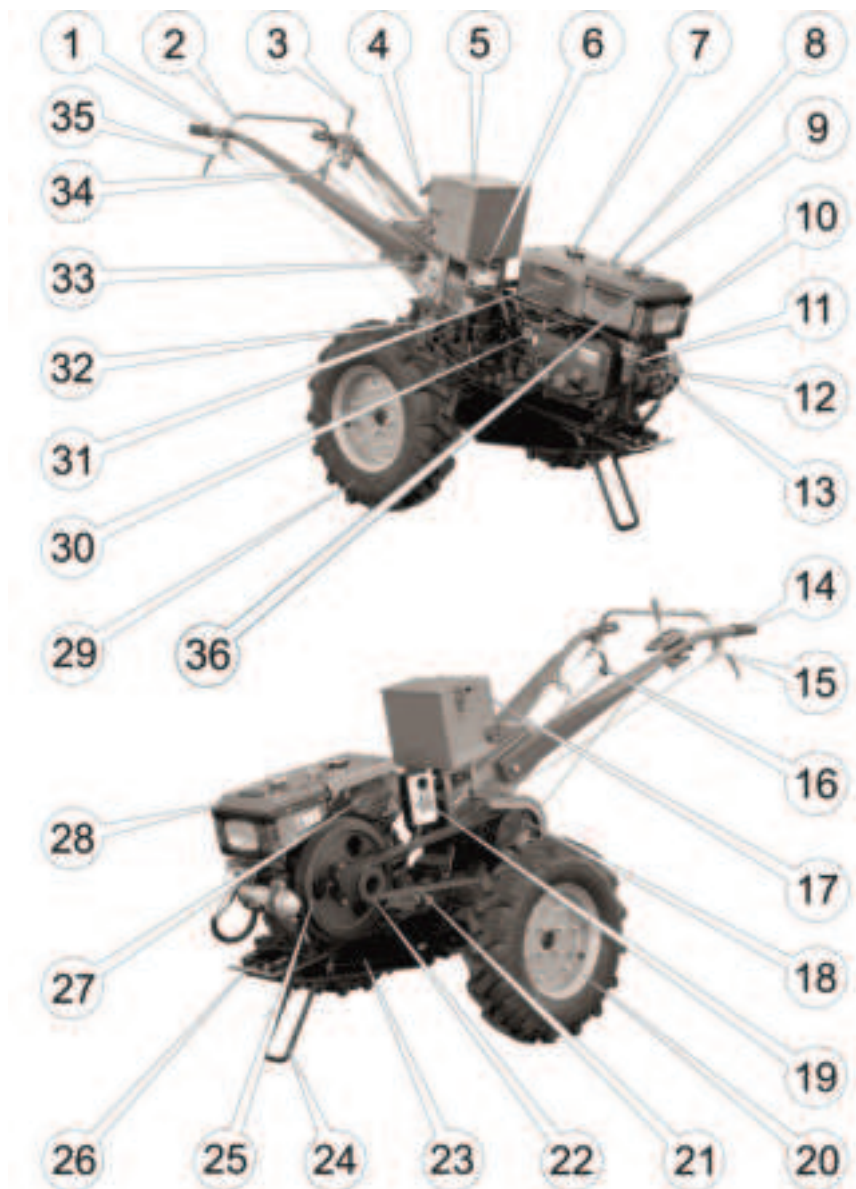
Рисунок 2. – Органи мотоблока МБ1080ДЕ-10
