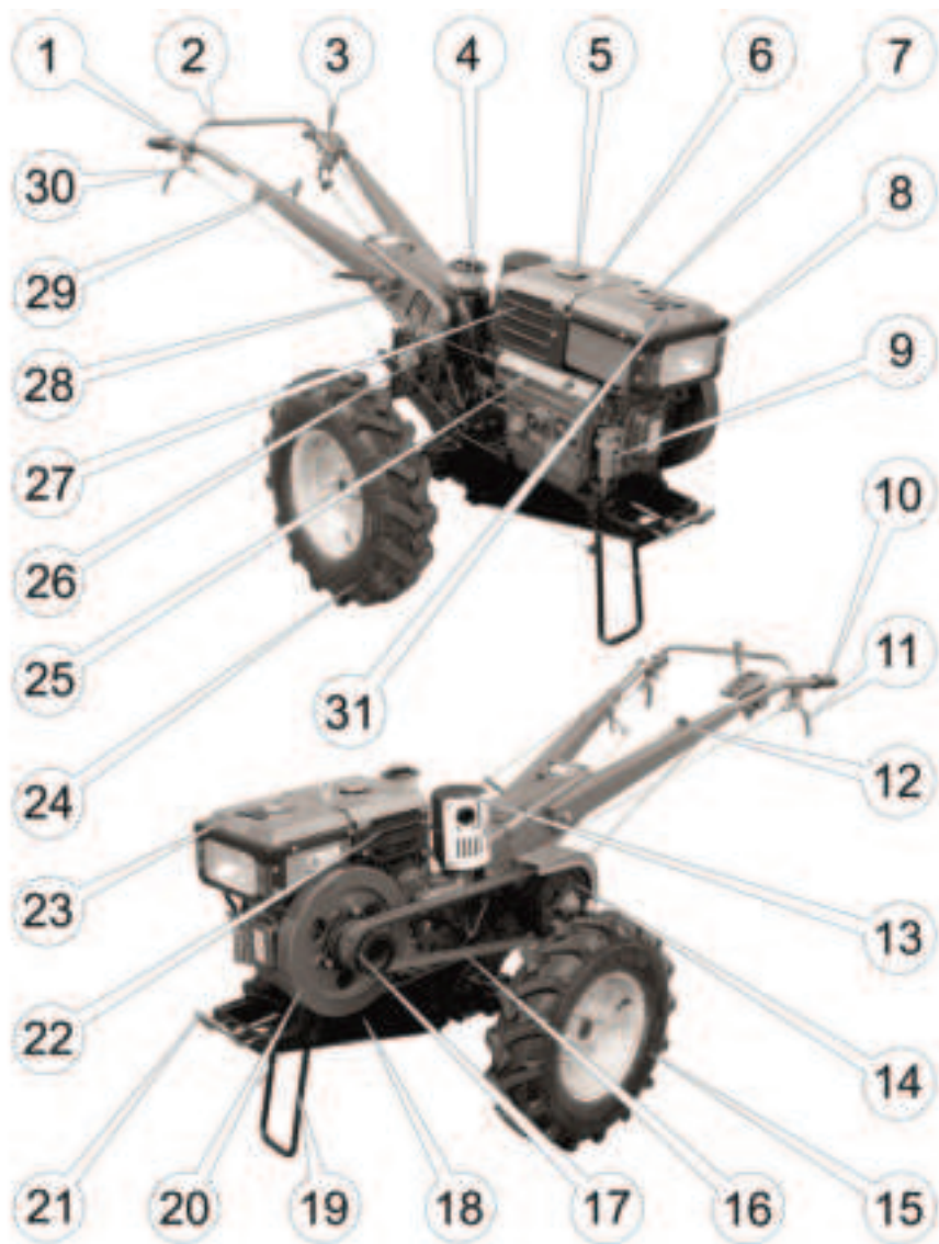
Рисунок 9. – Органи мотоблока МБ1012Д-10
