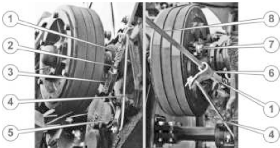
Рисунок 45. – Регулювання гальм
