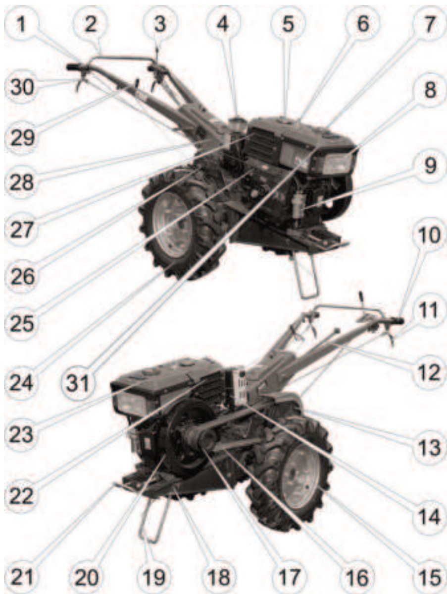
Рисунок 6. – Органи мотоблока МБ1010Д-10
