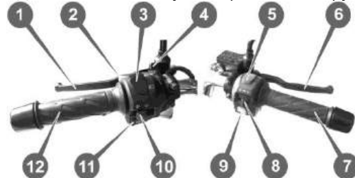
Рисунок 3.4. Блоки перемикачів
