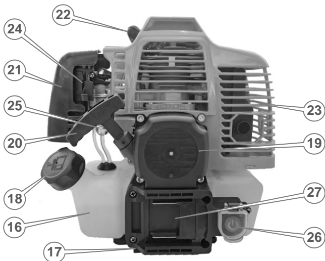
Рисунок 1. Загальний вигляд мотокоси ТМ «Vitals», серії «Vitals», моделі «BK 522n ES».
