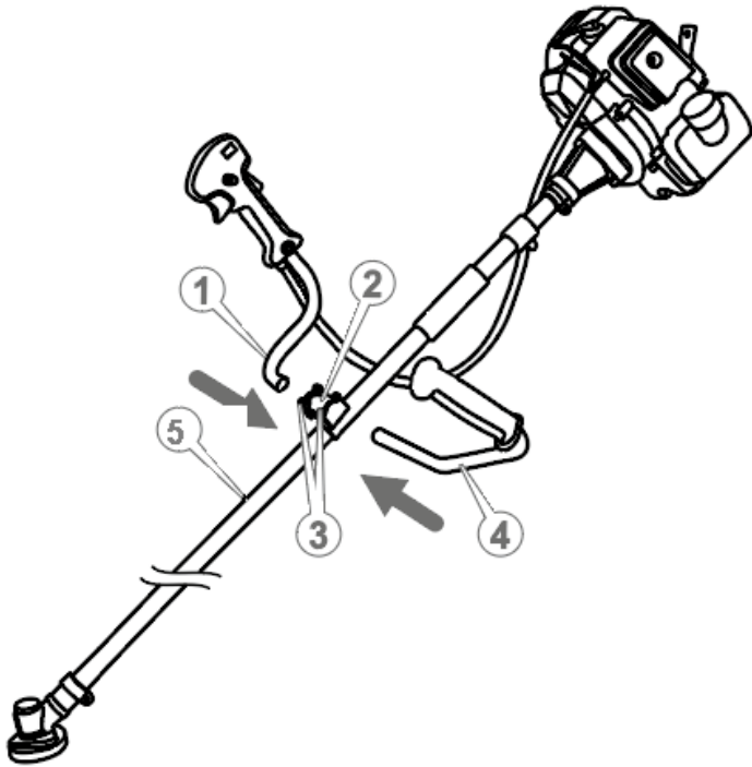
Рисунок 2. Схема встановлення руків'їв виробу.
