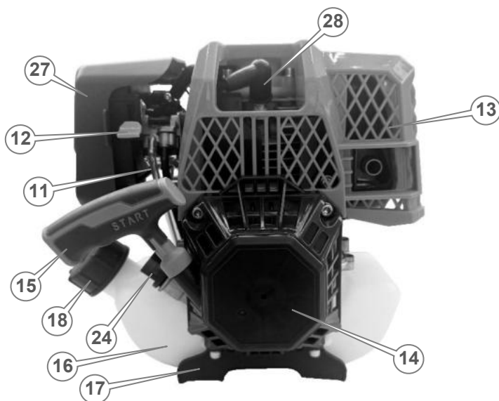
Рисунок 1. Загальний вигляд виробу.
