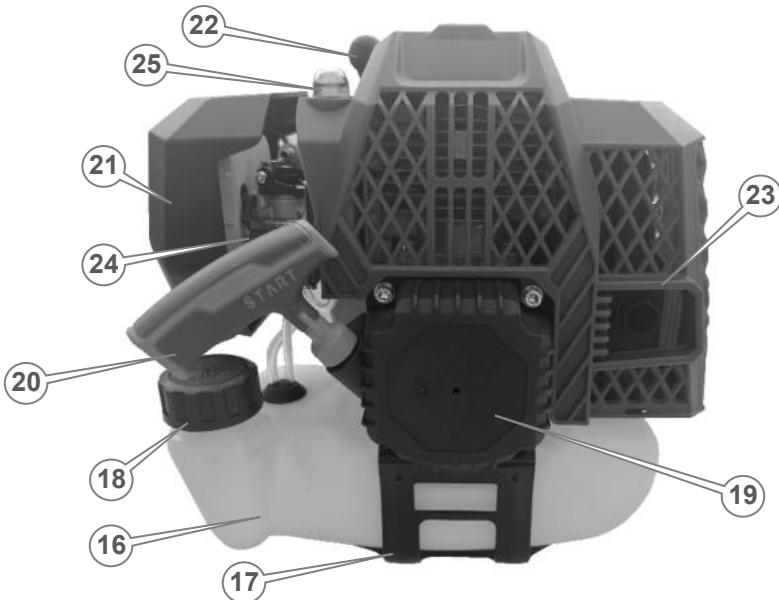
Рисунок 1. Загальний вигляд мотококси моделі «BK 523n».
