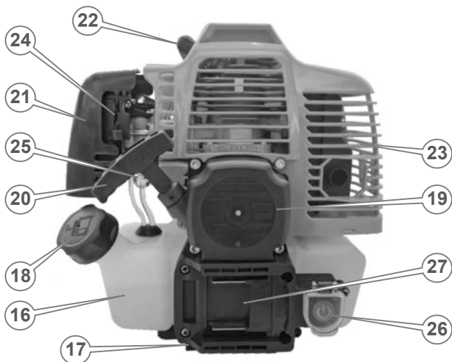
Рисунок 1. Загальний вигляд мотокози ТМ «Vitals», серії «Master», моделі «BK 523n ES».
