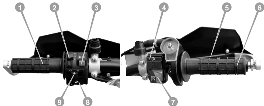
Рисунок 3. Права та ліва рукоятки керма
