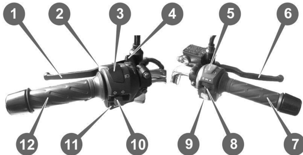
Рисунок 3.3. Блоки перемикачів
