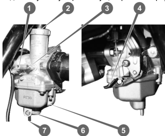
Рис. 6.6. Карбюратор
