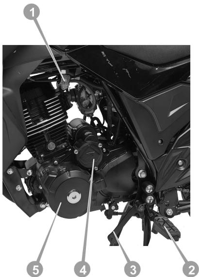
Рисунок 3.4. Двигун, вид зліва
