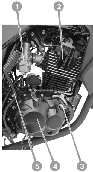
Рисунок 3.5. Двигун, вид справа
