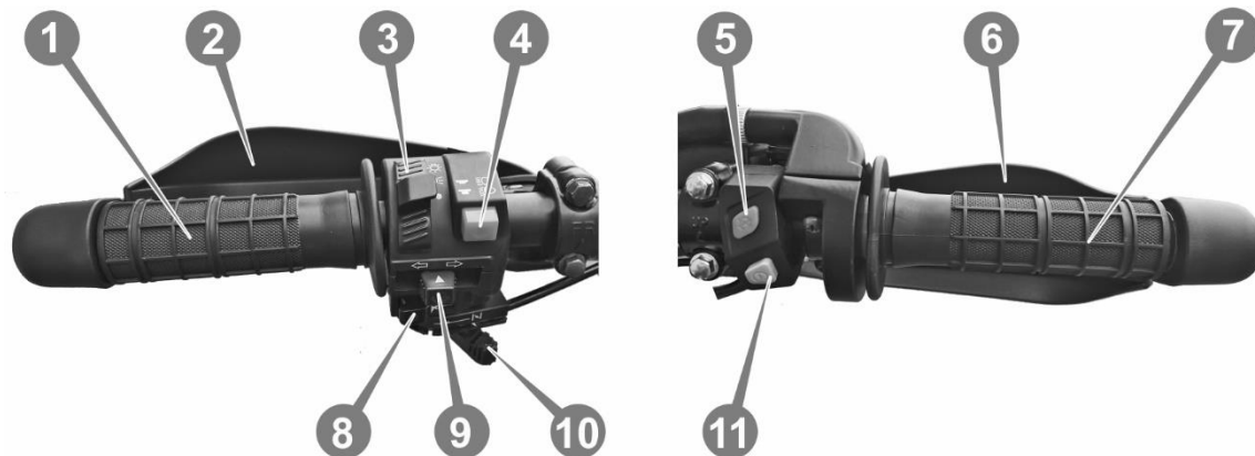
Рисунок 3.4. Блоки перемикачів.
