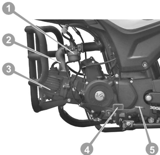
Рис. 4. Двигун, вид зліва.
