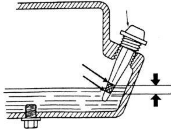
Рисунок 12. Перевірка рівня мастила у двигуні
