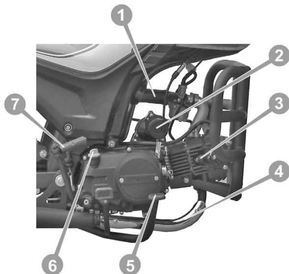
Рис. 5. Двигун, вид справа.
