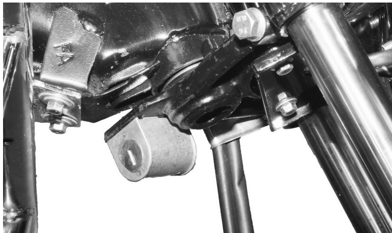
Рисунок 9. Замок блокування керма
