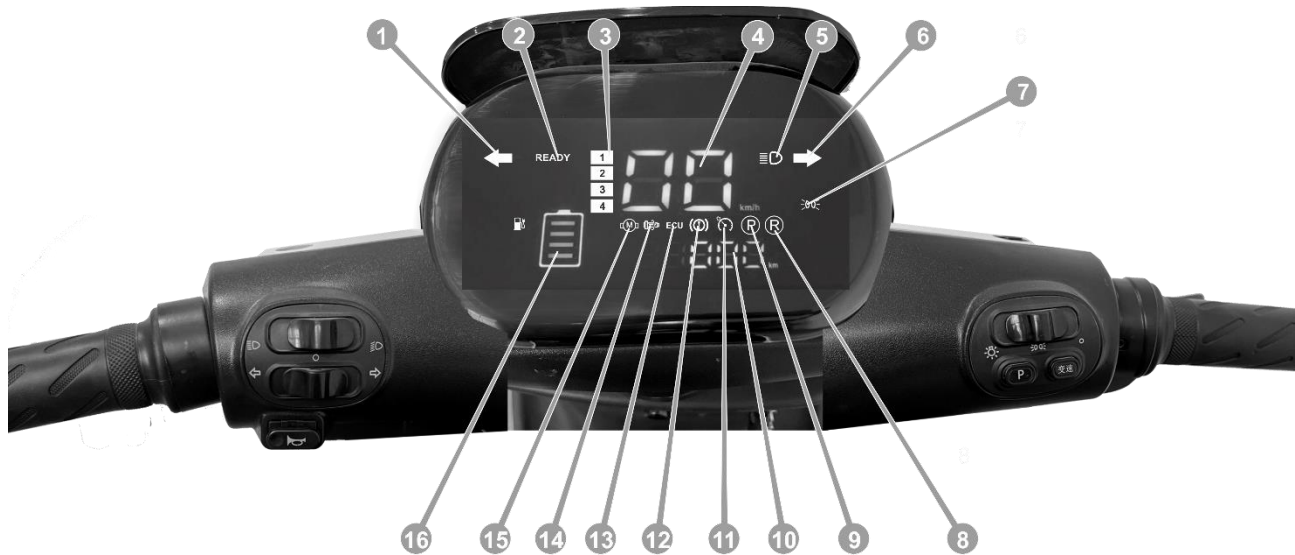
Рисунок 2.1. Панель приладів моделей електроскутера SP1500E-3
